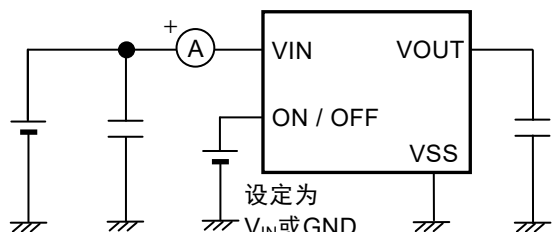
图9 测定电路2
