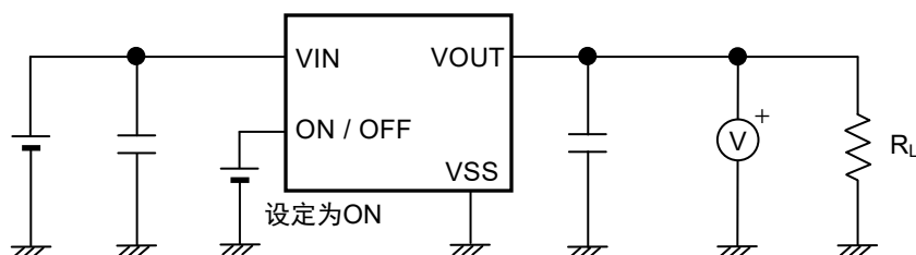
图13 测定电路6
