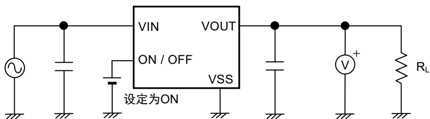
图12 测定电路5
