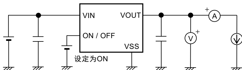
图8 测定电路1
