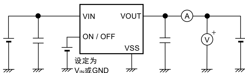
图10 测定电路3
