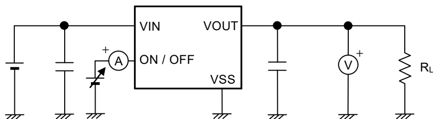
图11 测定电路4
