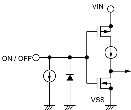
图14 S-1318系列A / C型
