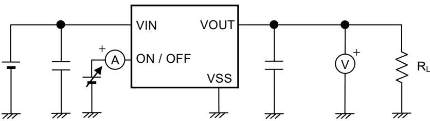
图10 测定电路4
