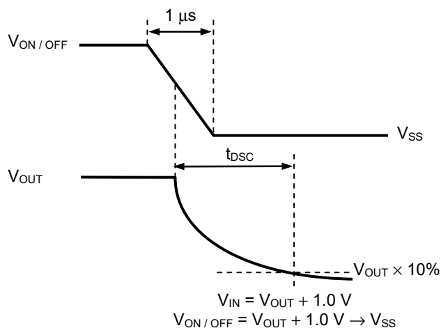
图18 放电时间的测定条件
