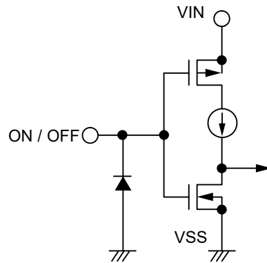
图17 S-1313xxxH系列B / D型
