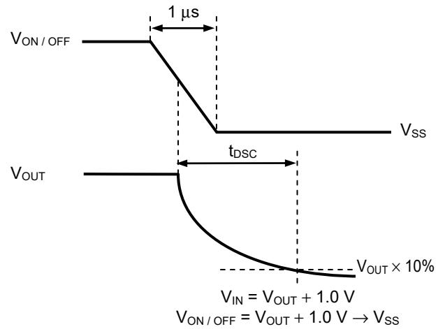
图21 放电时间的测定条件
