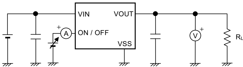
图14 测定电路4
