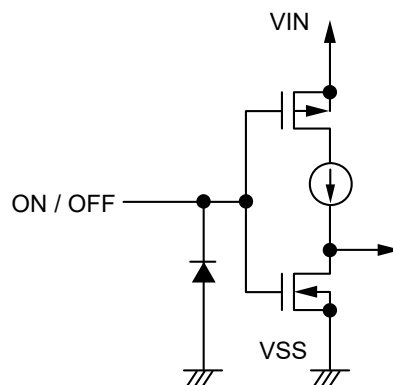
图19 S-1313系列B / D型
