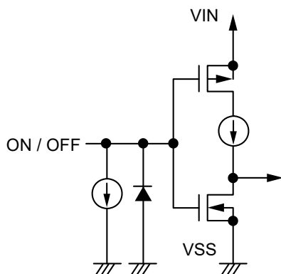
图18 S-1313系列A / C型
