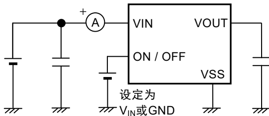
图12 测定电路2
