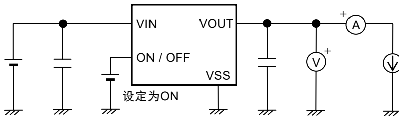
图11 测定电路1
