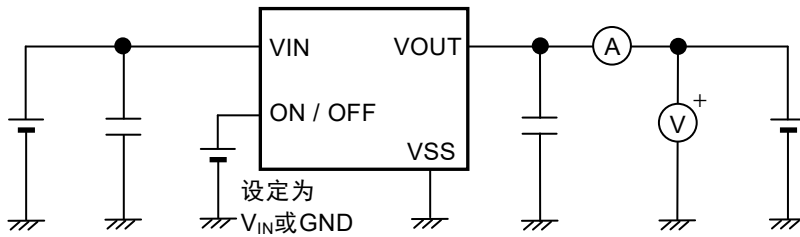
图13 测定电路3
