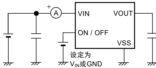
图12 测定电路2
