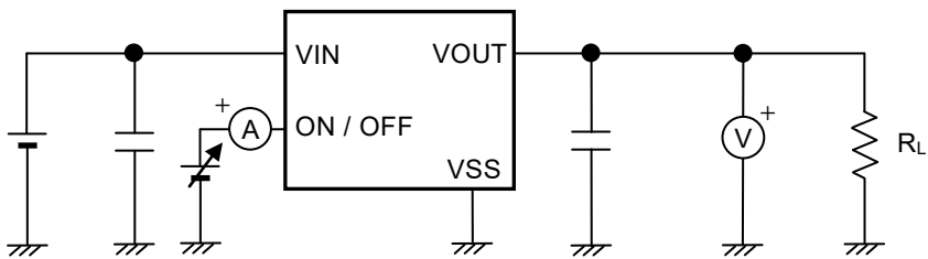
图14 测定电路4
