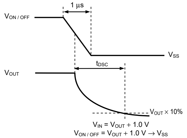
图23 放电时间的测定条件
