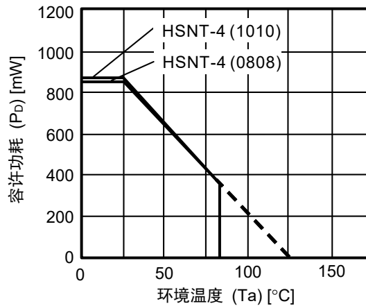
图10 封装容许功耗 (基板安装时)
