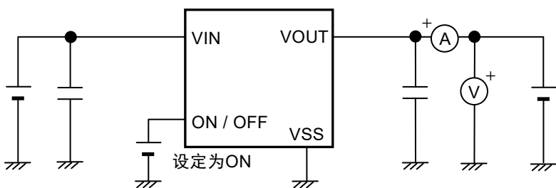
图7 测定电路3
