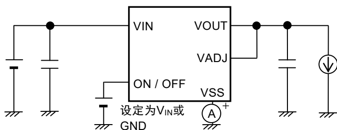
图12 测定电路8
