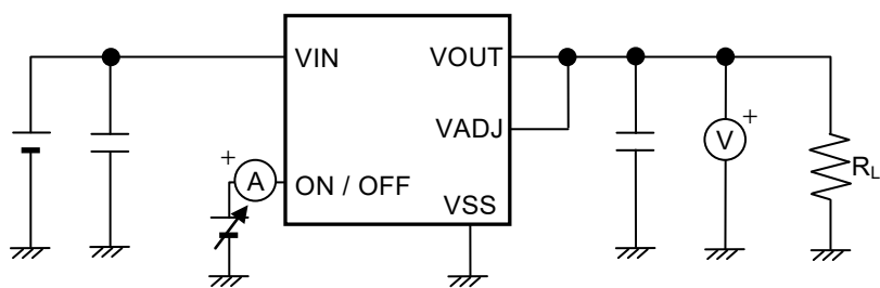
图14 测定电路10
