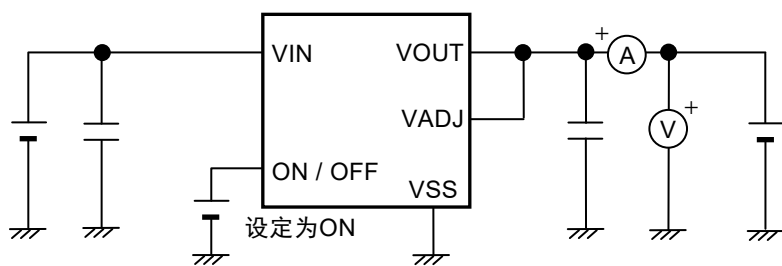
图13 测定电路9
