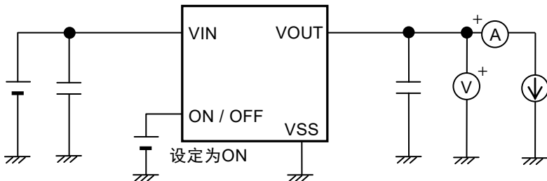
图5 测定电路1
