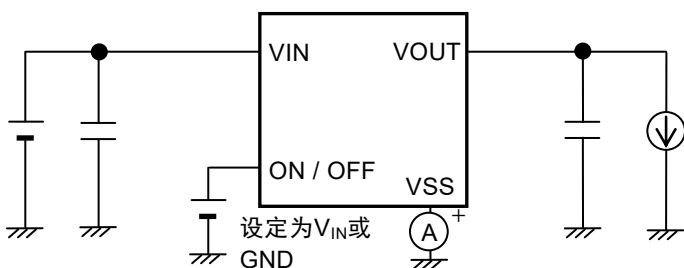
图6 测定电路2
