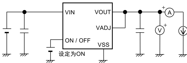
图11 测定电路7
