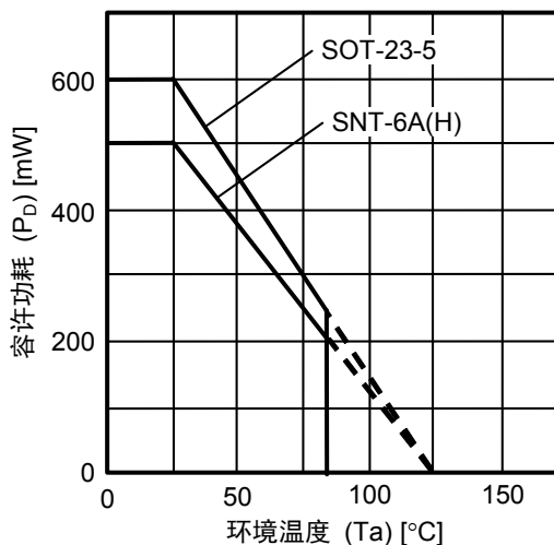
图4 封装容许功耗（基板安装时）
