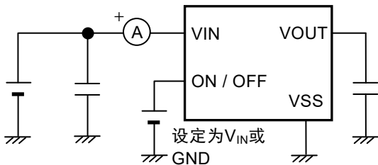
图6 测定电路2
