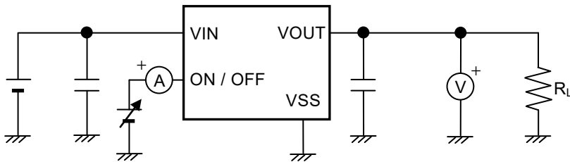
图8 测定电路4
