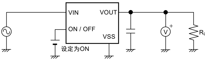
图9 测定电路5
