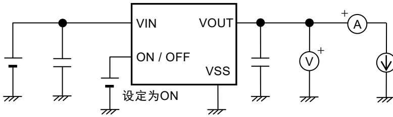
图5 测定电路1
