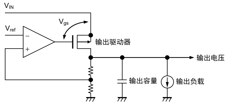
图13 电路图
