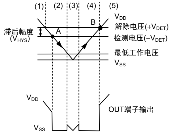
图18 工作说明图2
