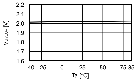
2.17 UVLO解除电压 ( V_{UVLO+} ) – 温度 ( T_a )
