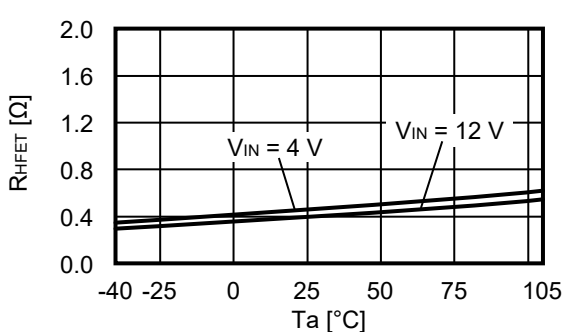
2.9 高侧功率MOS FET导通电阻 ( R_{HFET} ) – 温度 ( T_a )
