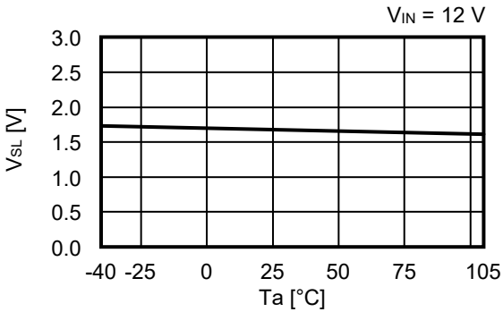
2. 15 低电位输入电压 (V SL ) – 温度 (Ta)
