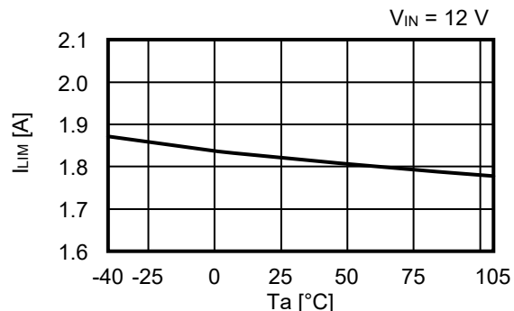
2.13 限制电流 ( I_{LIM} ) – 温度 ( T_a )
