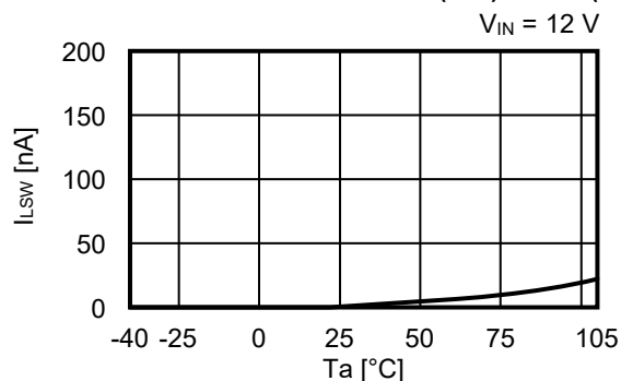
2.12 低侧功率MOS FET泄漏电流 ( I_{LSW} ) – 温度 ( T_a )
