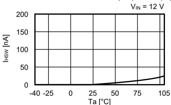
2.11 高侧功率MOS FET泄漏电流 ( I_{HSW} ) – 温度 ( T_a )
