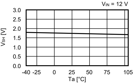
2. 14 高电位输入电压 (V SH ) – 温度 (Ta)
