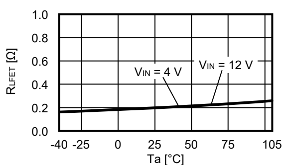
2.10 低侧功率MOS FET导通电阻 ( R_{LFET} ) – 温度 ( T_a )
