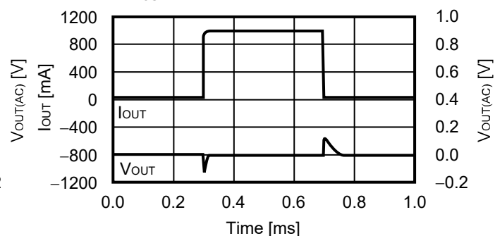
4.4.2 I_{OUT} = 10\text{ mA} \rightarrow 1000\text{ mA} \rightarrow 10\text{ mA}
