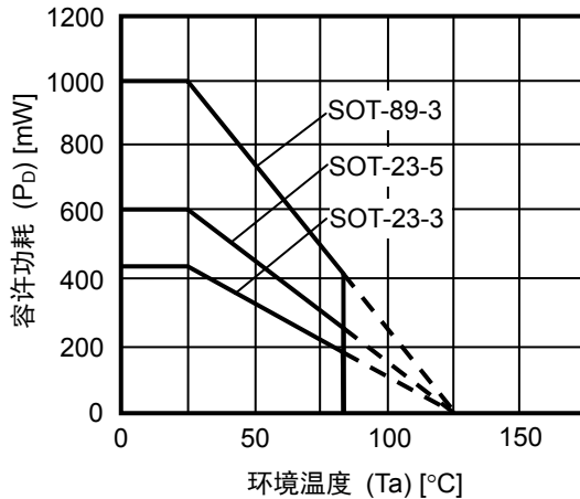
(1) 基板安装时
