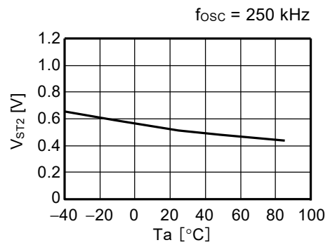
(14) 振荡开始电压( V_{ST2} ) - 温度( T_a )
