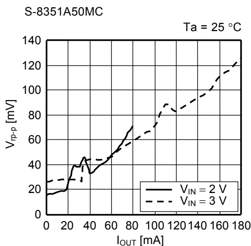
图16 输出电流( I_{OUT} ) - 纹波电压( V_{rp-p} )特性
