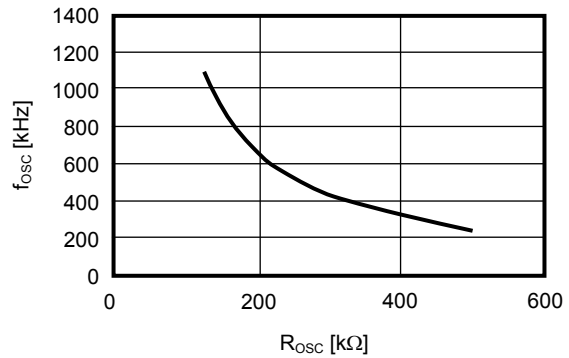
图12 R osc vs. f osc
