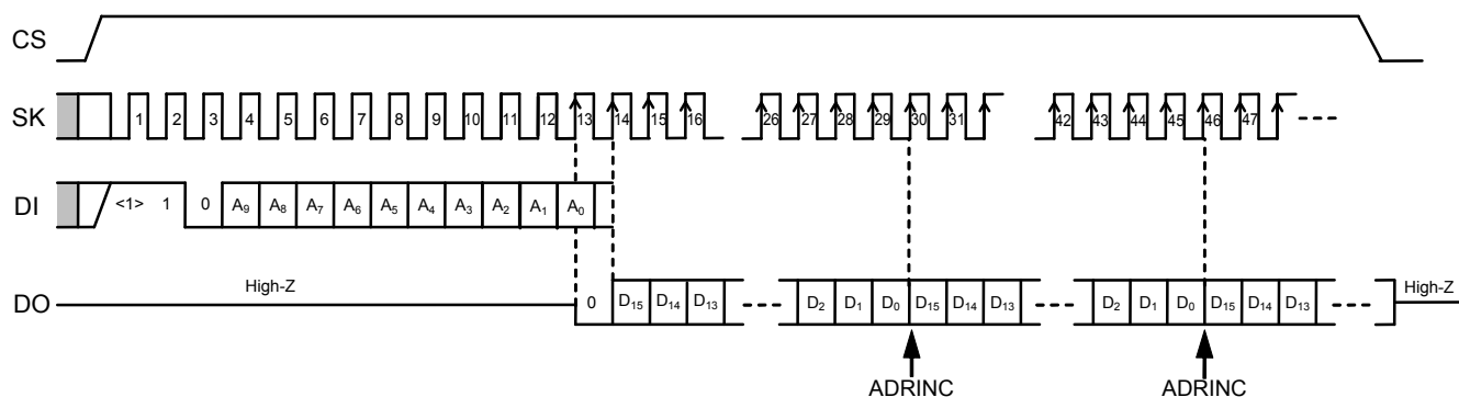
图5 读出定时
