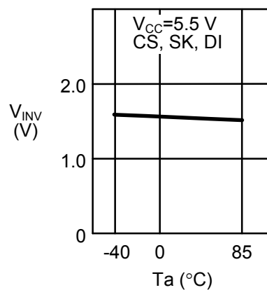
1. 28 输入反转电压 V_{INV} —周围温度 T_a
