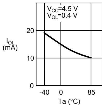
1. 25 低电位输出电流 I_{OL} —周围温度 T_a
