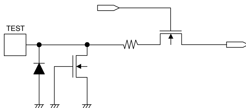
图16 TEST端子
