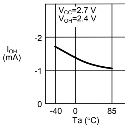
1. 23 高电位输出电流 I_{OH} —周围温度 T_a
