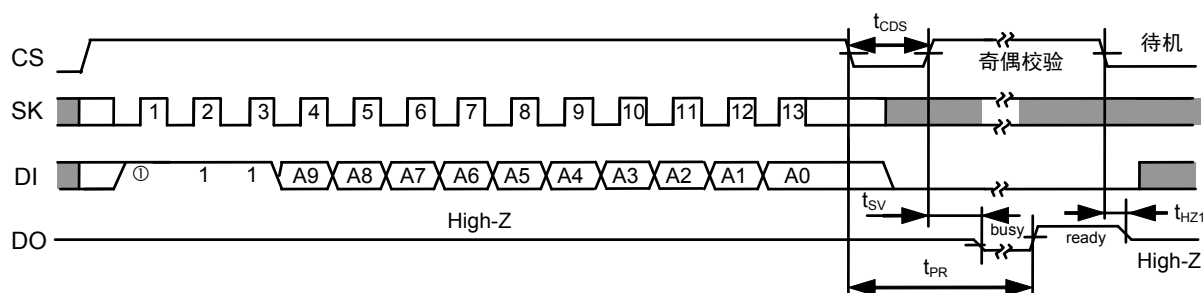
图7 数据删除定时
