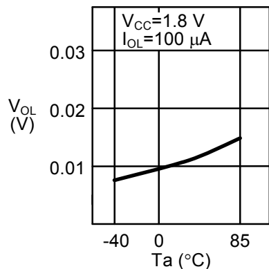
1. 21 低电位输出电压 V_{OL} —周围温度 T_a
