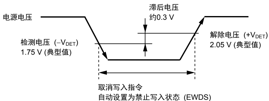
图11 低电源电压时的工作
