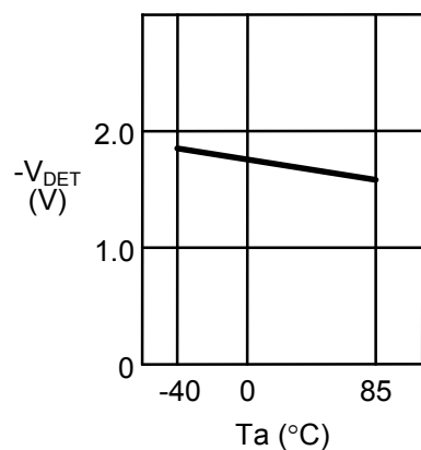
1. 29 低电源检测电压 -V_{DET} —周围温度 T_a
