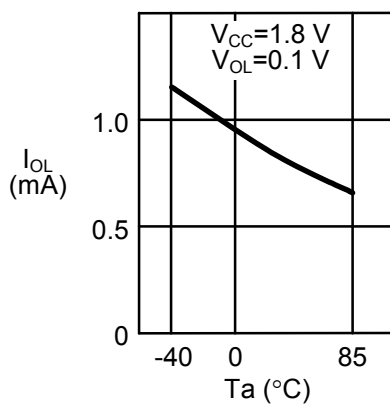
1. 26 低电位输出电流 I_{OL} —周围温度 T_a
