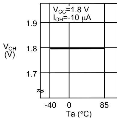
1. 19 高电位输出电压 V_{OH} —周围温度 T_a
