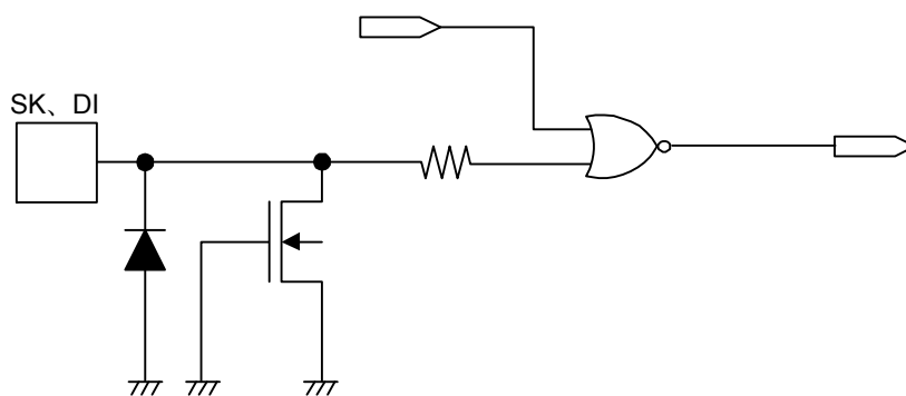
图15 SK、DI端子
