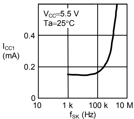
1.6 读出时消耗电流 I_{CC1} —时钟频率 f_{SK}
