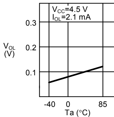
1. 20 低电位输出电压 V_{OL} —周围温度 T_a
