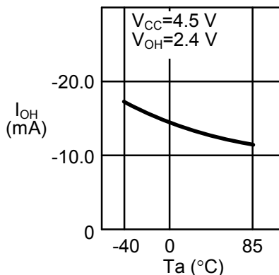
1. 22 高电位输出电流 I_{OH} —周围温度 T_a
