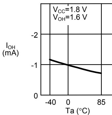
1. 24 高电位输出电流 I_{OH} —周围温度 T_a
