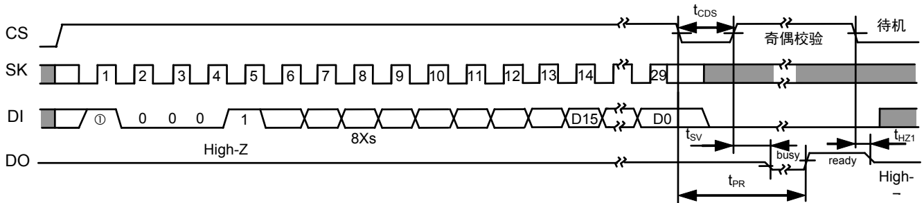
图8 全部写入定时
