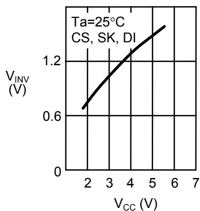
1. 27 输入反转电压 V_{INV} —电源电压 V_{CC}
