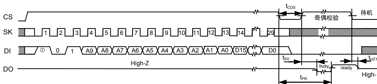
图6 数据写入定时
