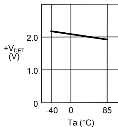
1. 30 低电源解除电压 +V_{DET} —周围温度 T_a
