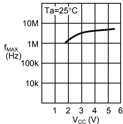
2.1 最大工作频率 f_{MAX} —电源电压 V_{CC}
