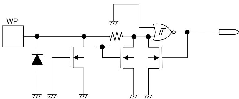
图21 WP端子
