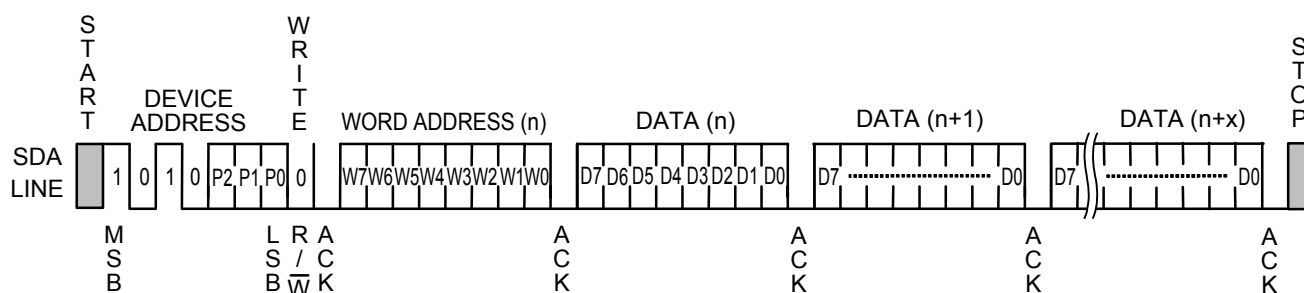
图12 页写入
