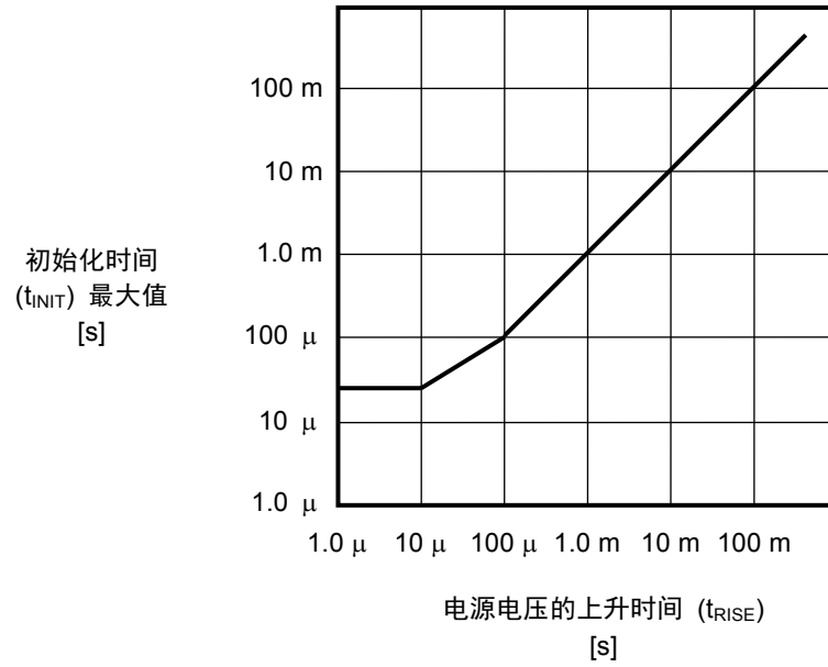
图25 S-24C16C的初始化时间
