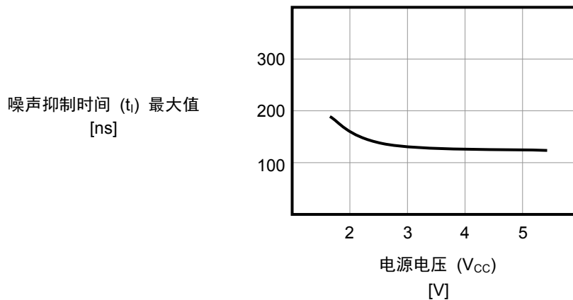
图27 SDA端子和SCL端子的噪声抑制时间
