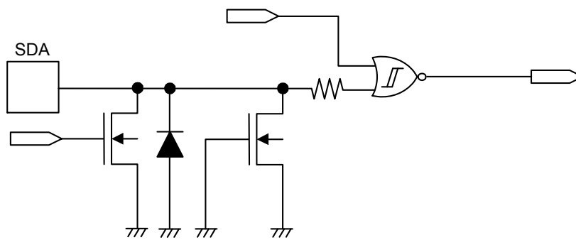
图20 SDA端子
