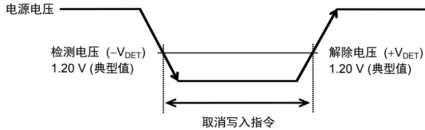
图18 低电源电压时的工作
