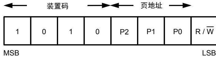
图10 装置地址
