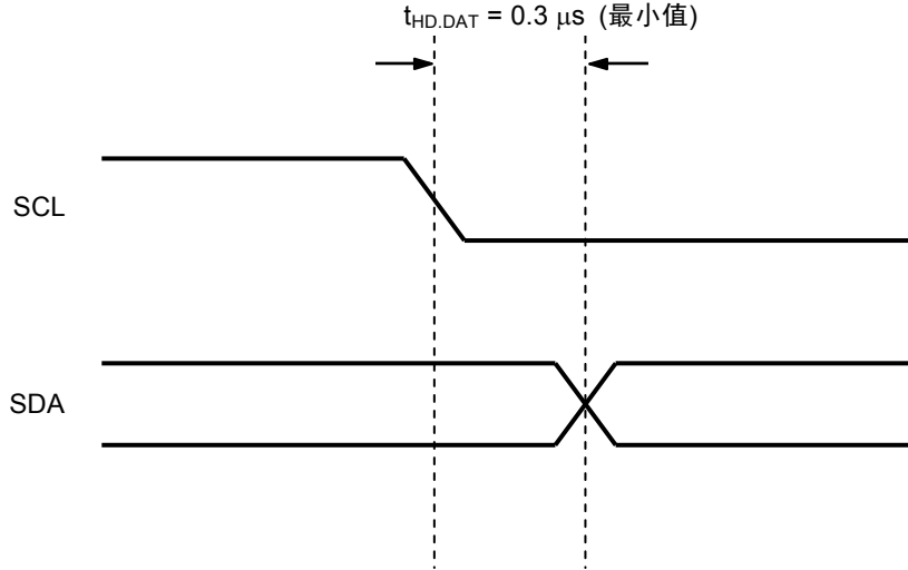
图26 S-24C16C的数据保持时间
