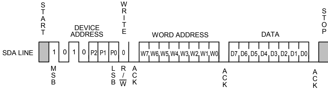
图11 字节写入
