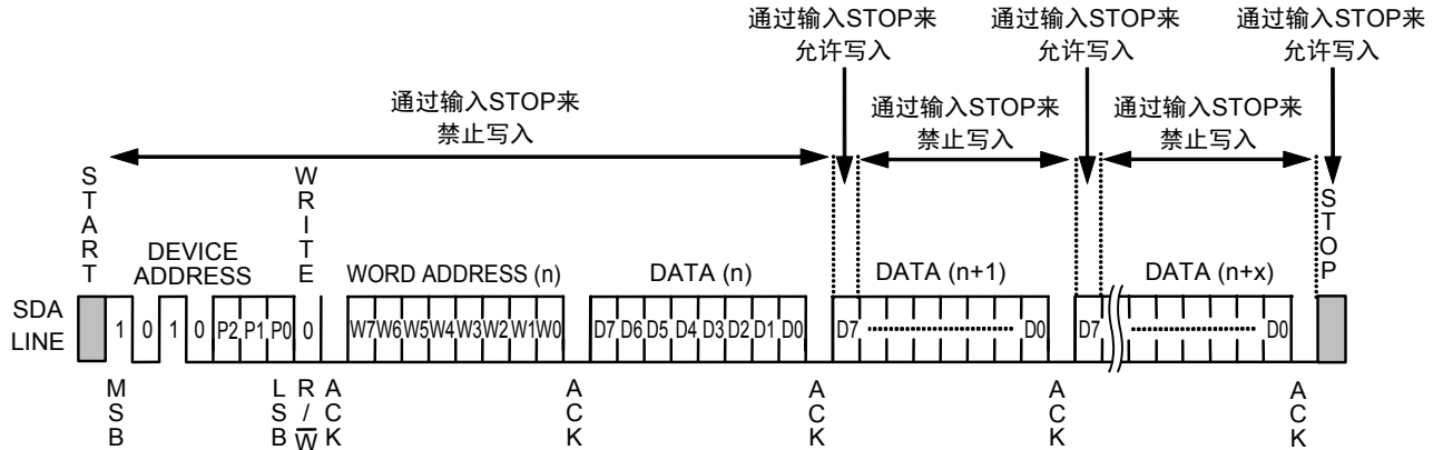
图 28 通过在写入过程中输入停止状态来执行写入工作
