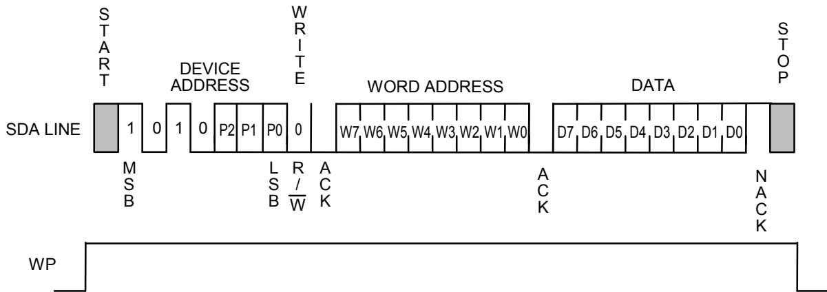
图13 写入保护
