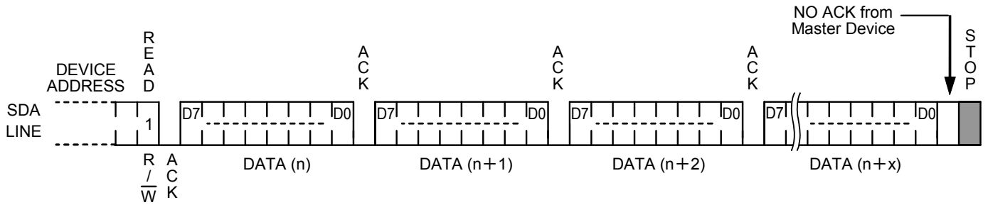
图17 顺序读出
