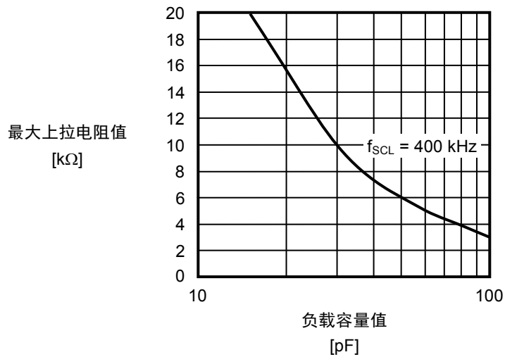
图6 输出负载
