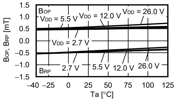
2.6.1 工作点、复位点 ( B_{OP} , B_{RP} ) – 温度 ( T_a )
