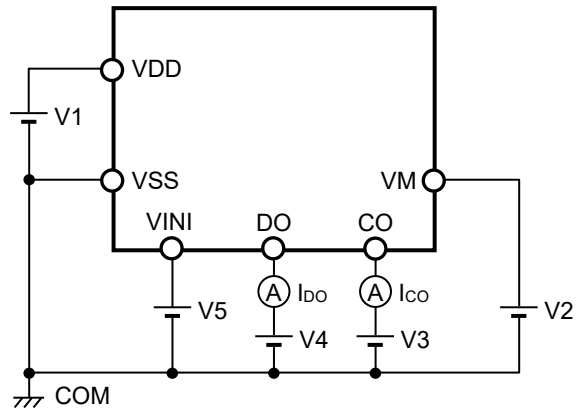
图6 测定电路4
