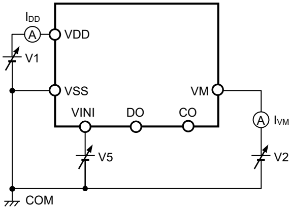
图5 测定电路3
