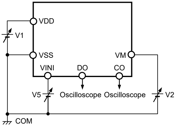
图7 测定电路5
