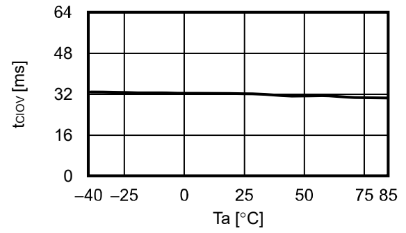
3.10 t_{CI0V} - T_a
