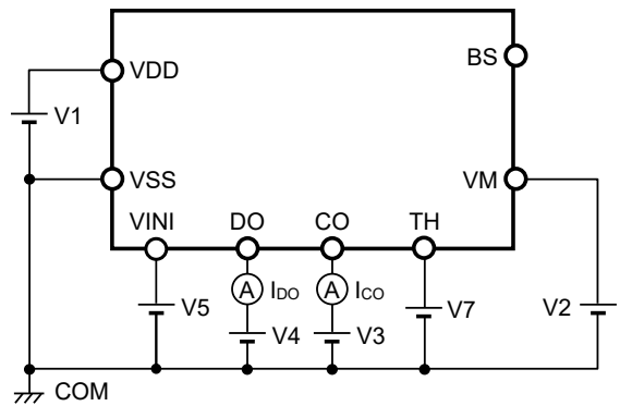
图6 测定电路4
