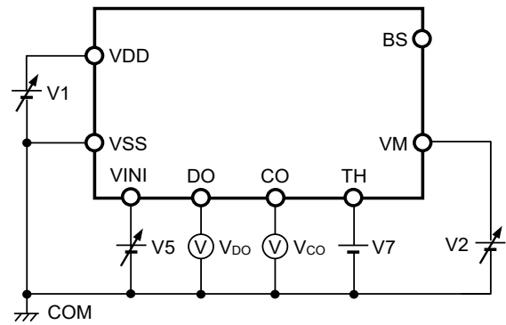
图4 测定电路2
