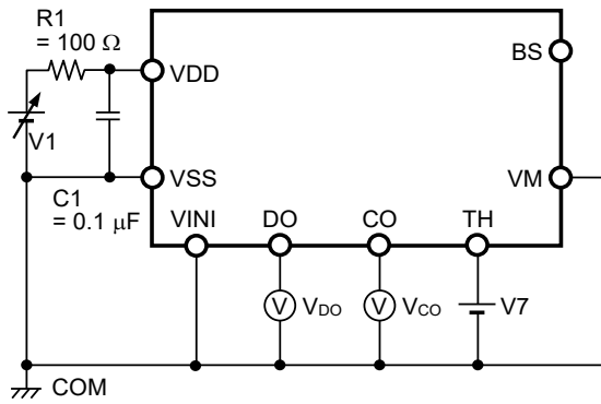
图3 测定电路1
