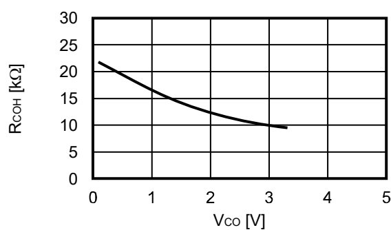
4. 1 R_{COH} - V_{CO}
