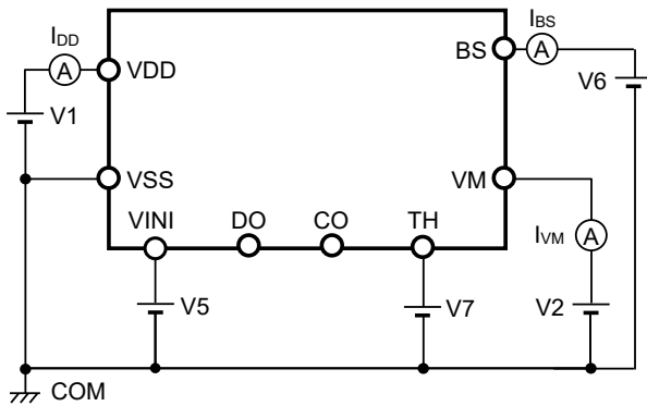
图5 测定电路3
