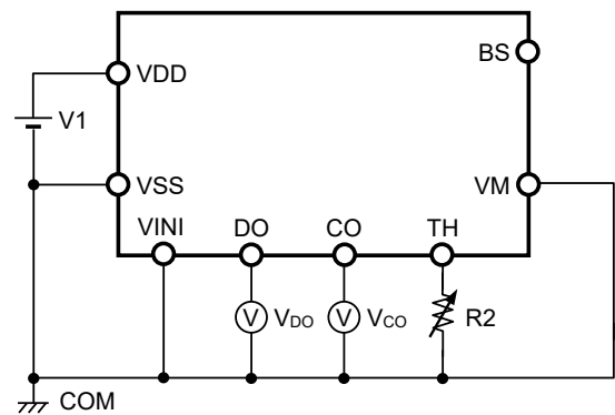
图8 测定电路6
