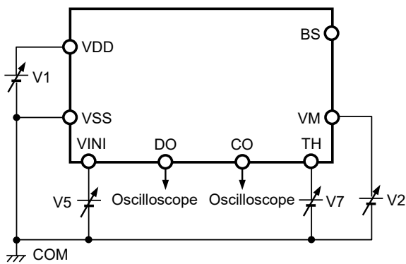
图7 测定电路5
