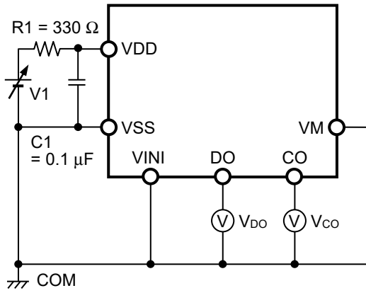
图3 测定电路1
