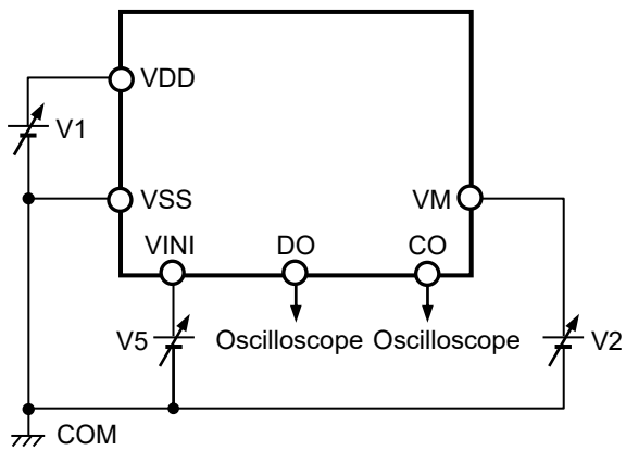
图7 测定电路5
