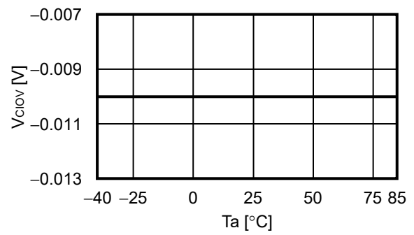
2.10 V_{CLOV} - T_a
