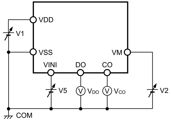
图4 测定电路2
