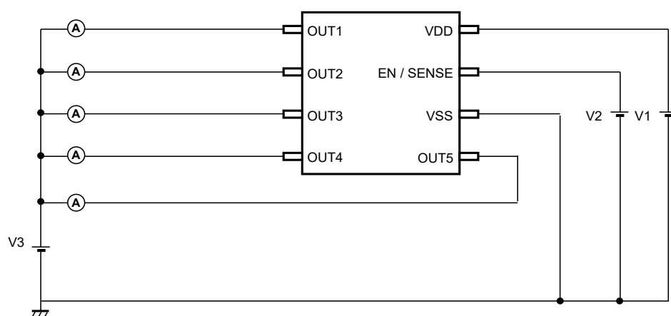
图4 测定电路1
