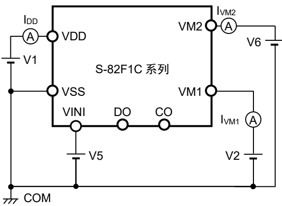
图5 测定电路3
