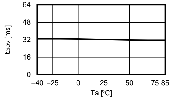
3.10 t_{CLOV} - T_a
