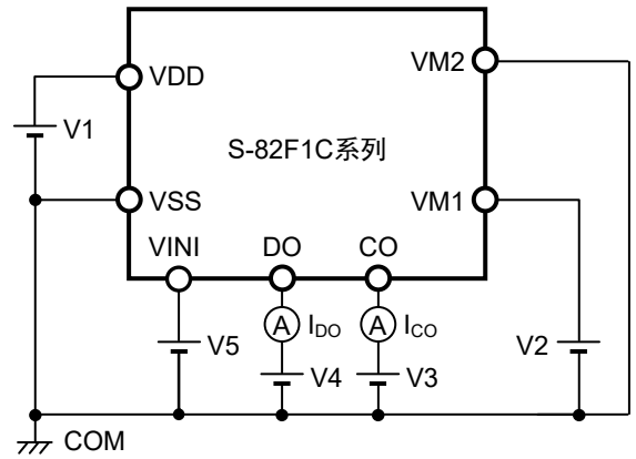
图6 测定电路4
