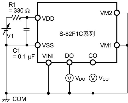
图3 测定电路1
