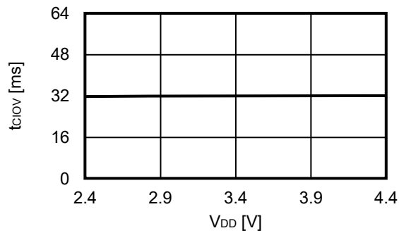
3.9 t_{CLOV} - V_{DD}
