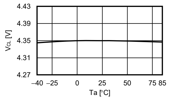
2.2 V_{cl} - T_a
