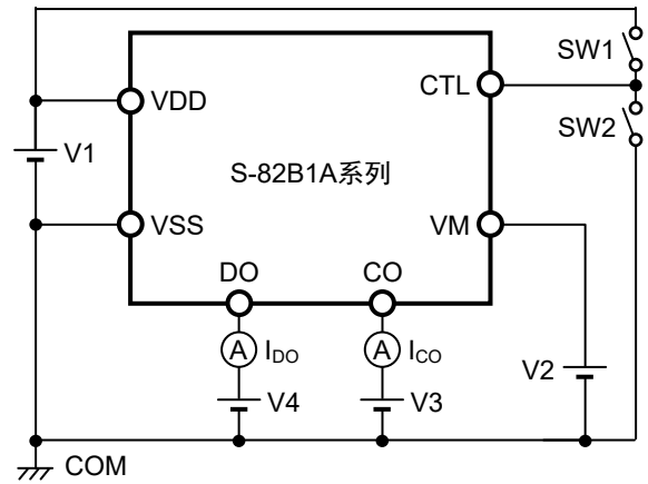
图7 测定电路4
