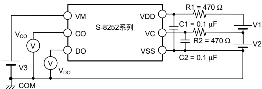
图5 测定电路1
