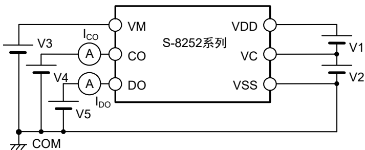
图8 测定电路4
