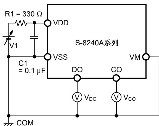
图6 测定电路1
