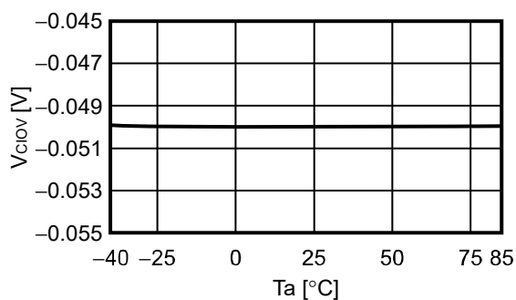
2.7 V_{CIOV} - T_a
