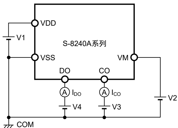
图9 测定电路4
