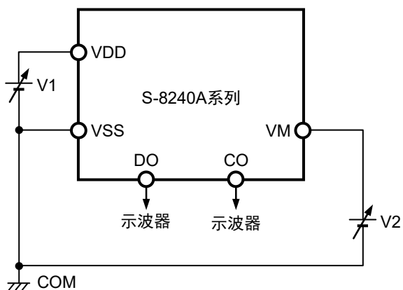
图10 测定电路5
