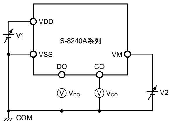
图7 测定电路2
