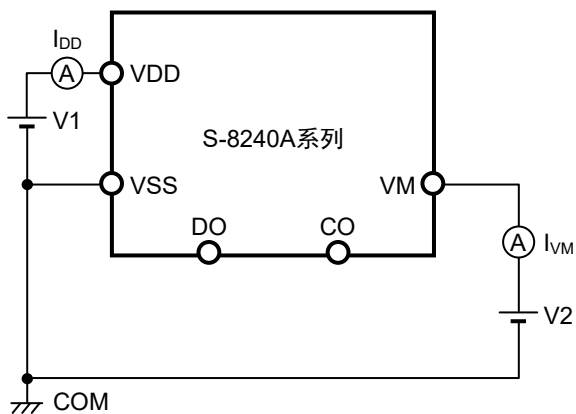
图8 测定电路3
