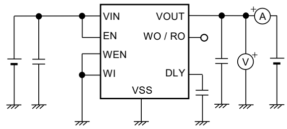
图10 测定电路2
