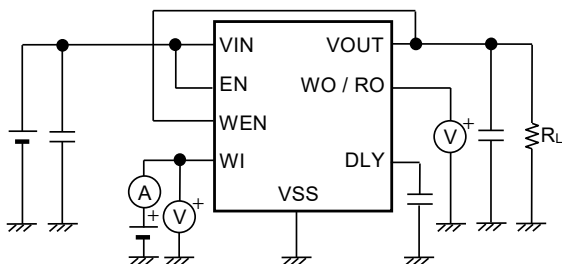
图15 测定电路7
