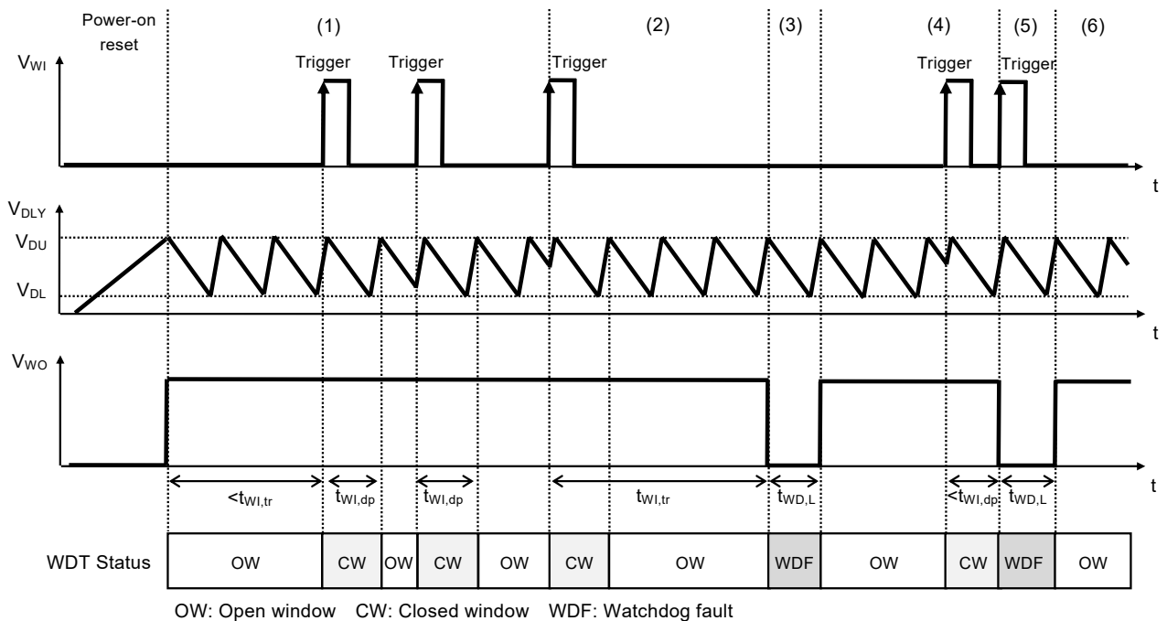
图24 看门狗定时器部分的时序图
