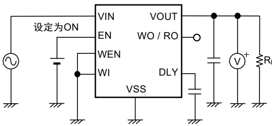
图11 测定电路3
