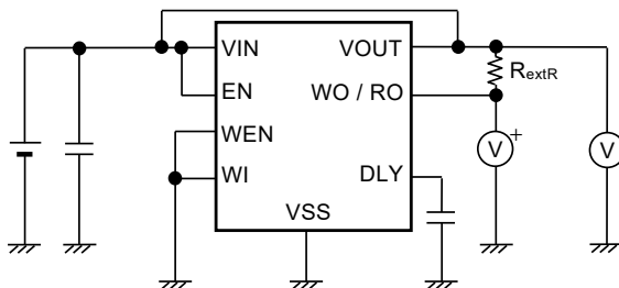
图13 测定电路5
