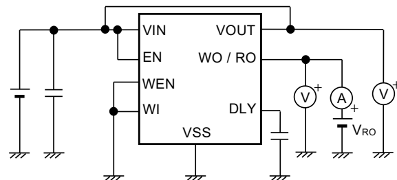
图14 测定电路6
