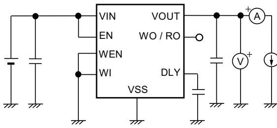
图9 测定电路1
