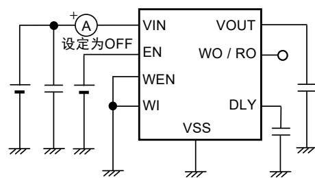
图18 测定电路10
