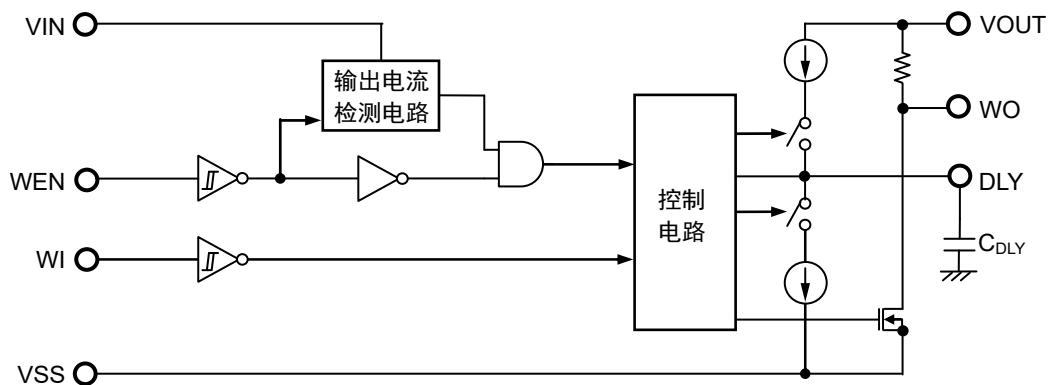
图26 看门狗定时器部分的工作说明图
