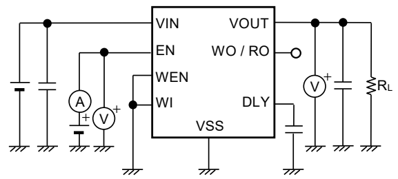
图12 测定电路4
