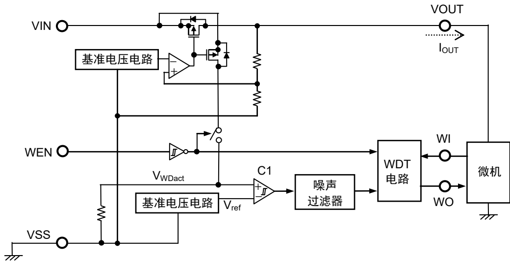
图27 输出电流检测电路工作说明图
