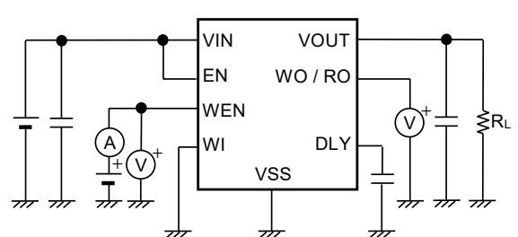
图16 测定电路8
