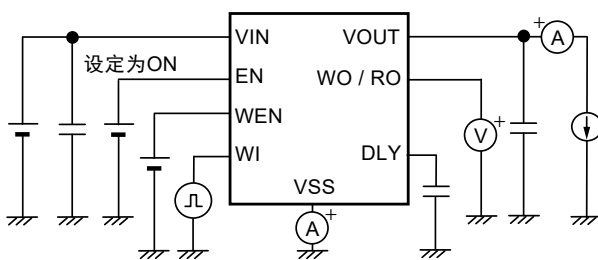
图17 测定电路9
