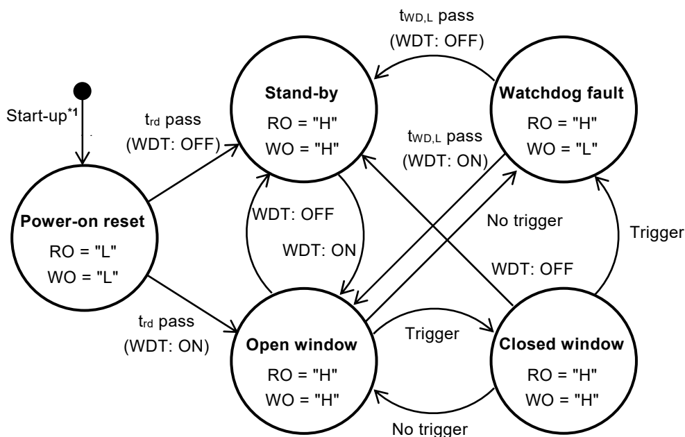
图25 看门狗定时器部分的状态迁移图
