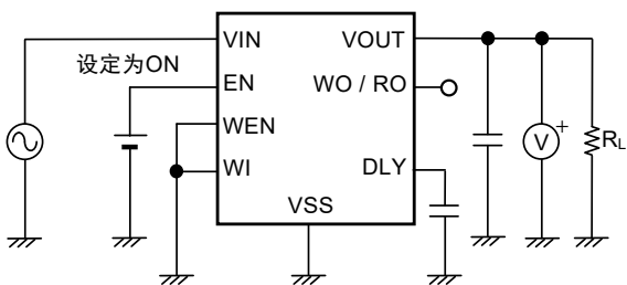
图11 测定电路3
