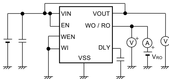
图14 测定电路6
