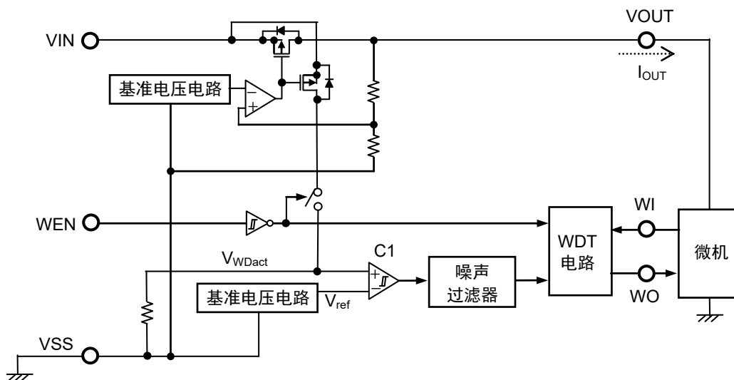
图27 输出电流检测电路工作说明图
