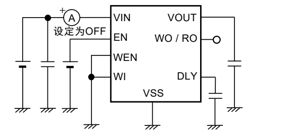
图18 测定电路10
