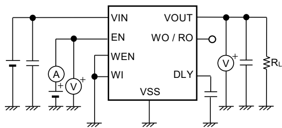
图12 测定电路4
