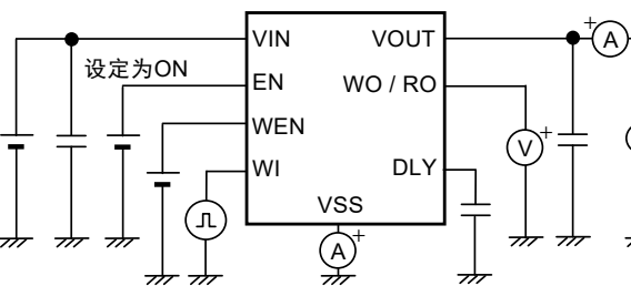
图17 测定电路9
