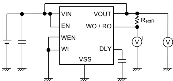
图13 测定电路5
