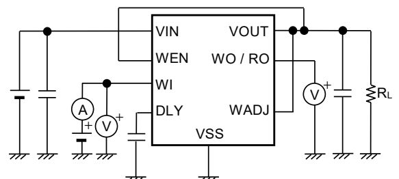
图19 测定电路8
