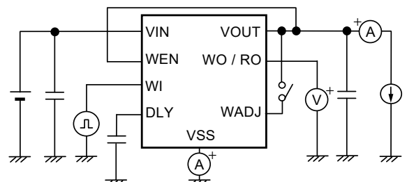
图21 测定电路10
