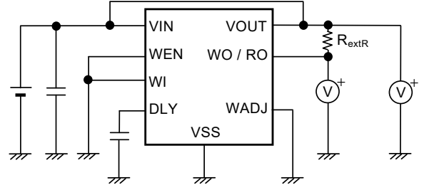
图15 测定电路4
