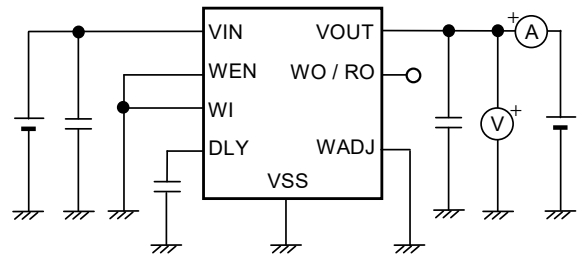
图13 测定电路2
