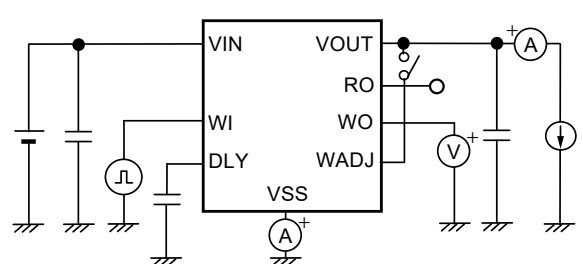
图31 测定电路10
