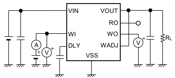
图29 测定电路8
