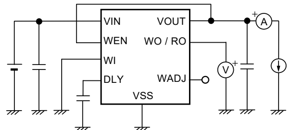
图17 测定电路6
