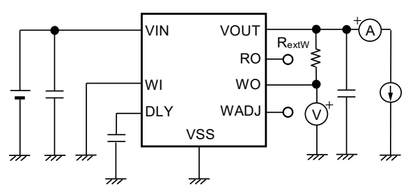
图27 测定电路6
