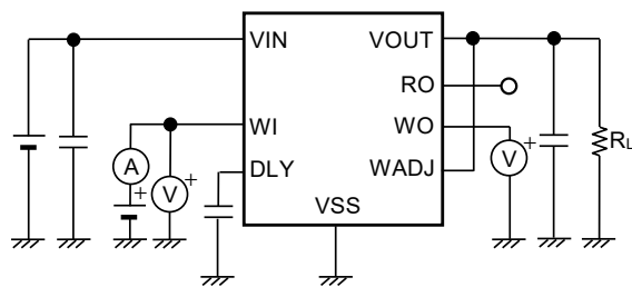
图27 测定电路8
