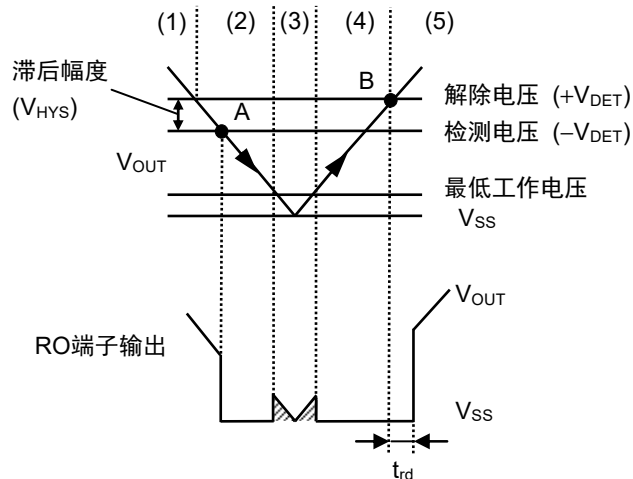
图34 检测器部分的时序图
