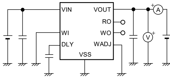
图21 测定电路2
