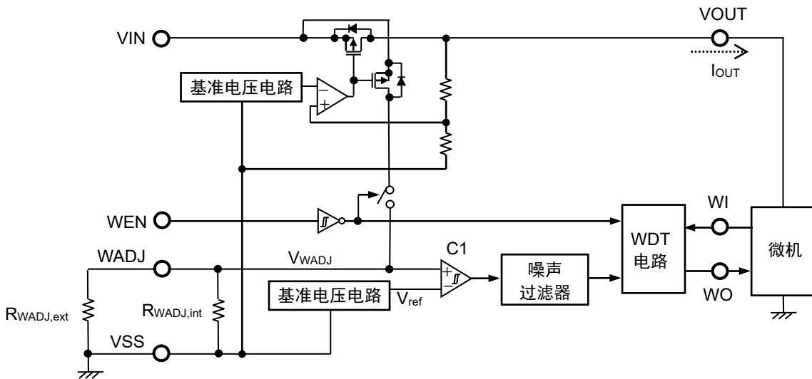
图37 输出电流检测电路工作说明图
