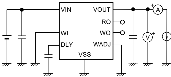
图20 测定电路1
