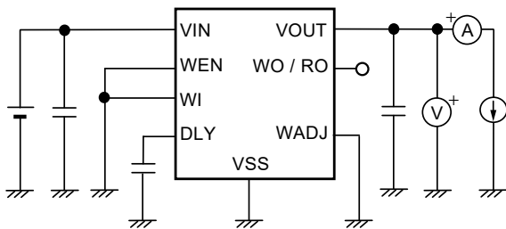
图10 测定电路1
