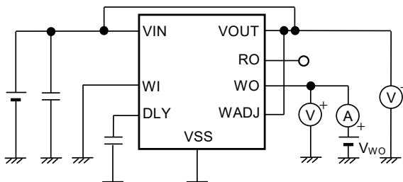
图28 测定电路9
