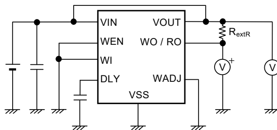
图13 测定电路4
