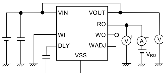
图24 测定电路5
