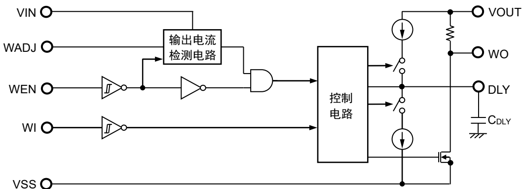
图36 看门狗定时器部分的工作说明图
