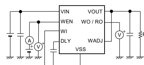
图18 测定电路9
