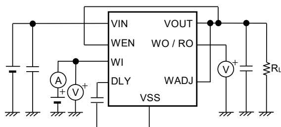
图17 测定电路8
