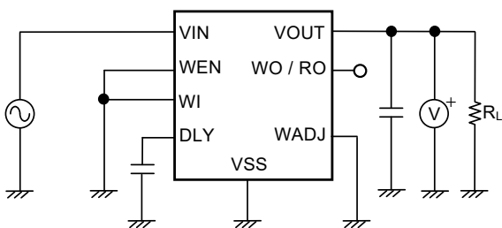
图12 测定电路3
