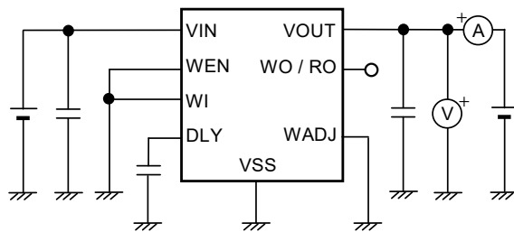
图11 测定电路2
