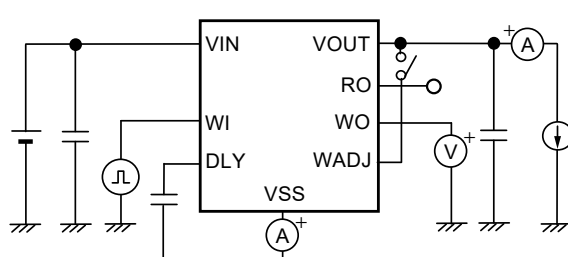
图29 测定电路10
