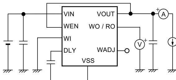
图15 测定电路6
