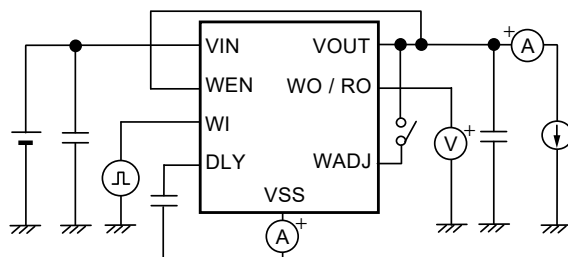
图19 测定电路10
