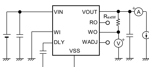
图25 测定电路6
