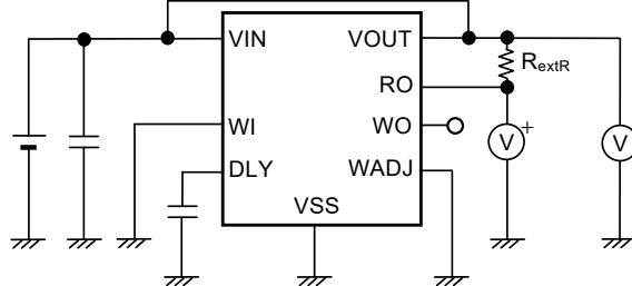
图23 测定电路4
