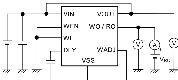
图14 测定电路5
