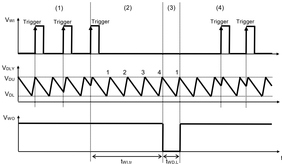
图35 看门狗定时器部分的时序图
