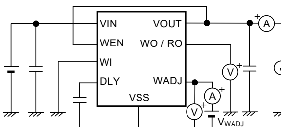
图16 测定电路7
