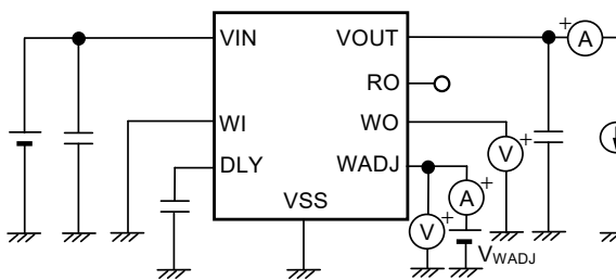
图26 测定电路7
