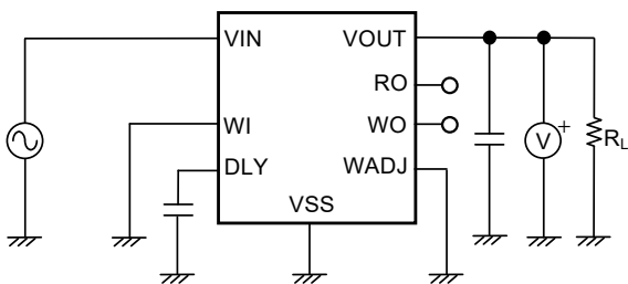
图22 测定电路3
