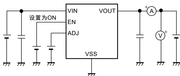
图13 测定电路9
