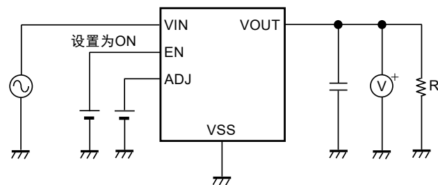
图12 测定电路8
