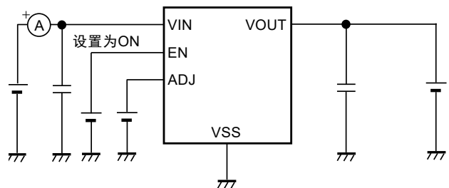
图8 测定电路4
