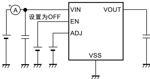
图9 测定电路5
