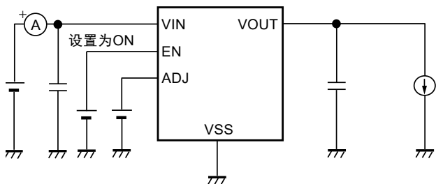
图7 测定电路3
