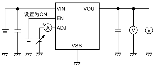
图11 测定电路7
