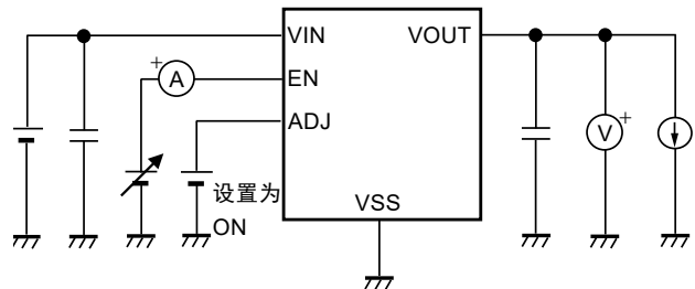
图10 测定电路6
