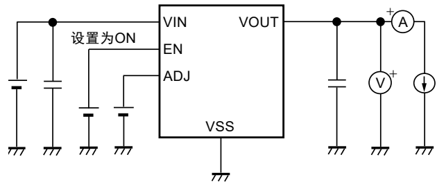
图6 测定电路2
