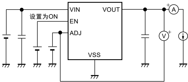
图5 测定电路1
