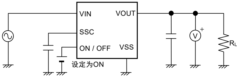
图7 测定电路5
