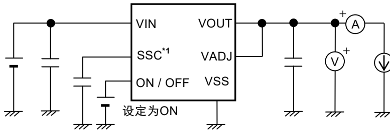
图17 测定电路8
