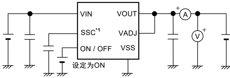
图19 测定电路10
