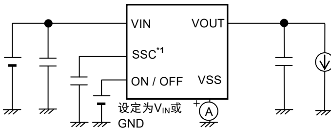
图11 测定电路2
