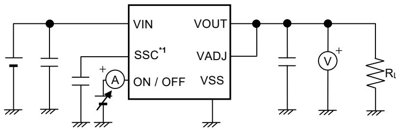
图20 测定电路11
