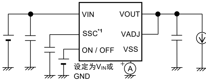
图18 测定电路9
