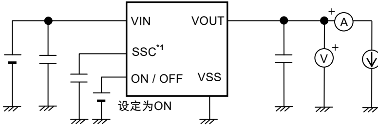
图10 测定电路1
