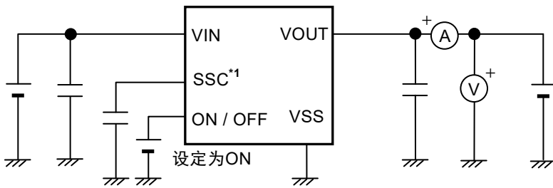
图12 测定电路3
