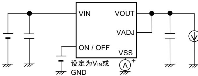
图12 测定电路8
