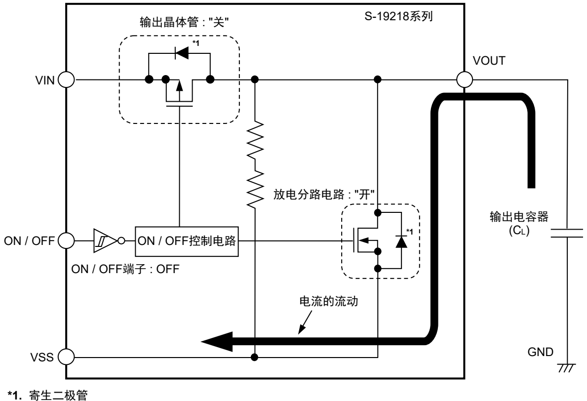
图22
