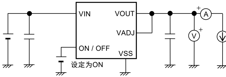
图11 测定电路7
