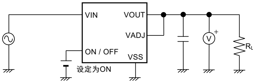
图15 测定电路11
