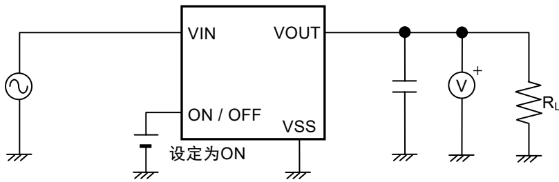
图9 测定电路5
