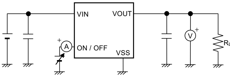
图8 测定电路4
