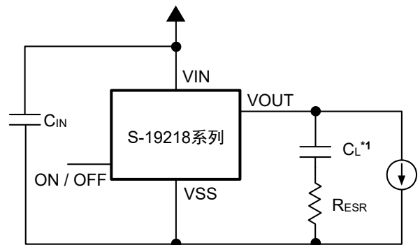
图25
