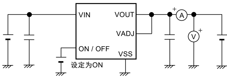
图13 测定电路9
