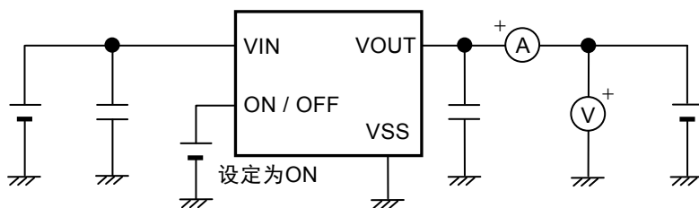
图7 测定电路3
