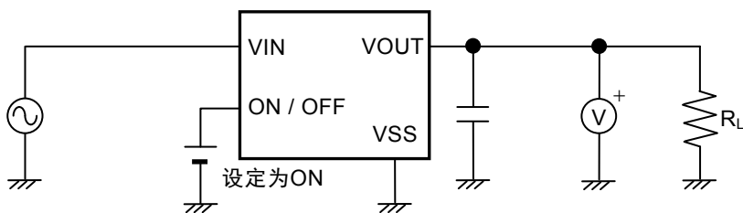
图9 测定电路5
