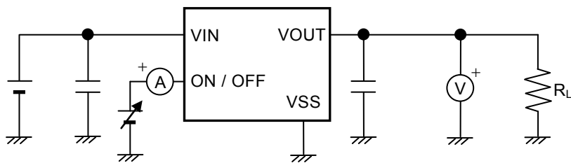
图8 测定电路4
