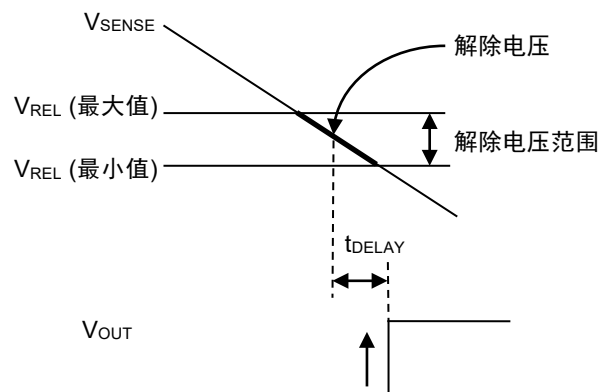
图12 解除电压
