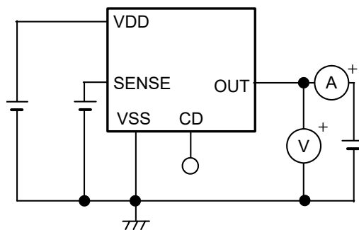
图7 测定电路2
