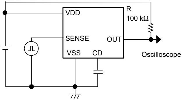
图8 测定电路3
