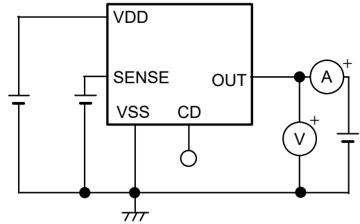
图7 测定电路2
