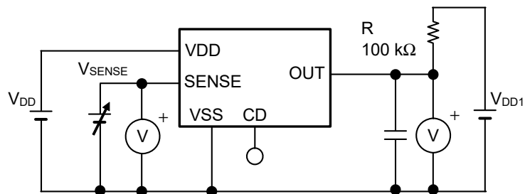
图21 响应时间的测定电路
