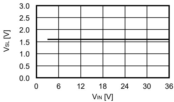
1.11 低电位输入电压 ( V_{SL} ) – 输入电压 ( V_{IN} )
