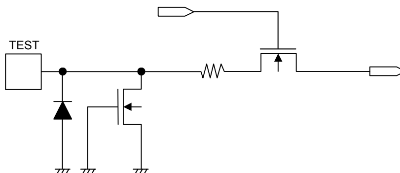
图18 TEST端子
