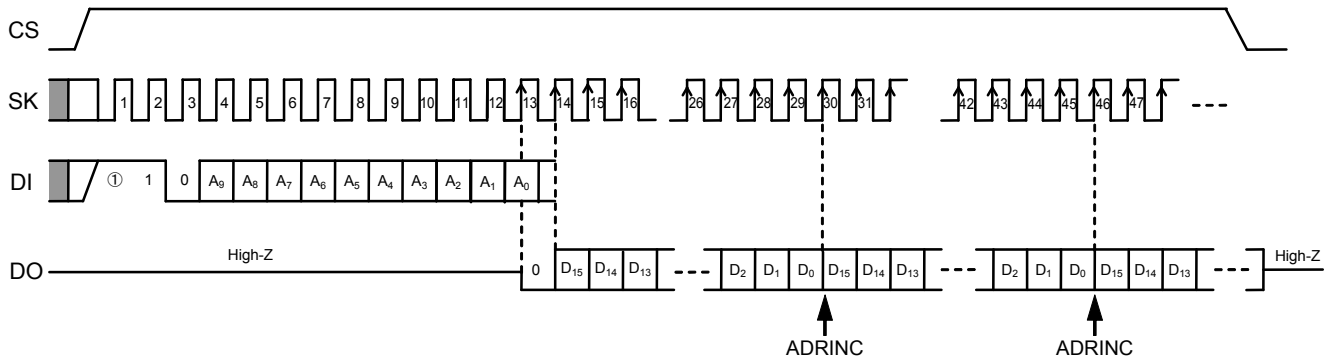
图 6 读出定时
