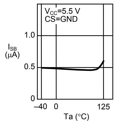
1. 11 待机时消耗电流 I_{SB} —周围温度 T_a
