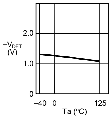
1. 36 低电源解除电压 +V_{DET} —周围温度 T_a
