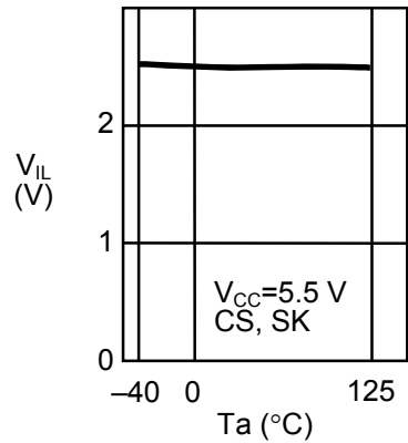
1. 32 低电位输入电压 V_{IL} —周围温度 T_a
