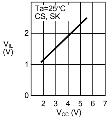
1. 31 低电位输入电压 V_{IL} —电源电压 V_{CC}
