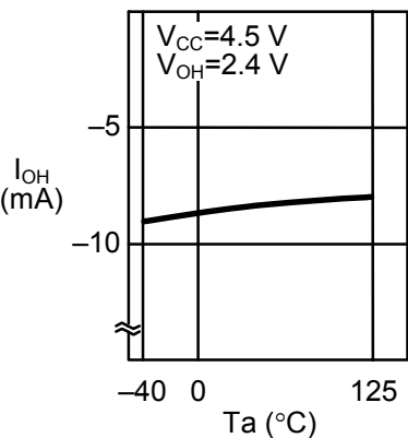
1. 22 高电位输出电流 I_{OH} —周围温度 T_a
