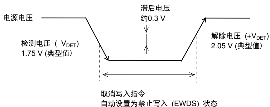
图18 低电源电压时的工作
