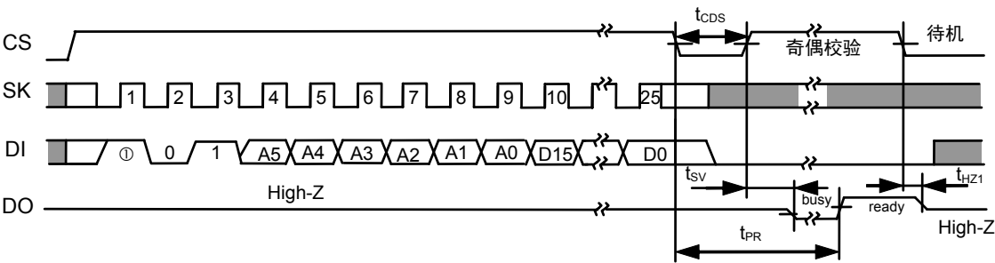
图8 数据写入定时 (S-93A46A)
