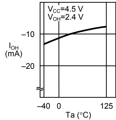
1. 22 高电位输出电流I OH —周围温度Ta
