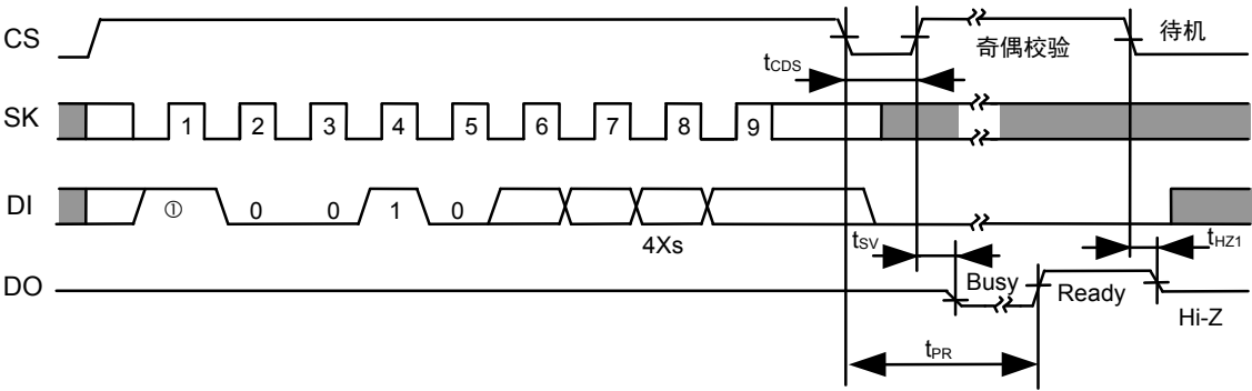
图14 全部删除定时 (S-93A46A)
