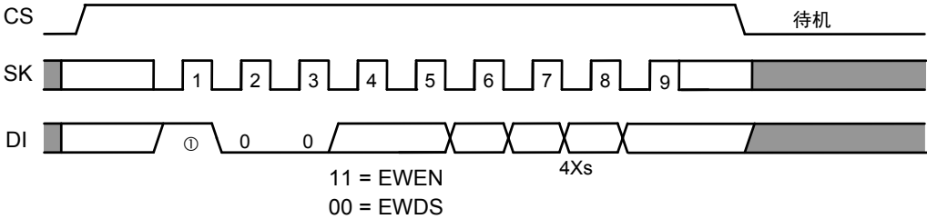
图16 允许或禁止写入定时 (S-93A46A)
