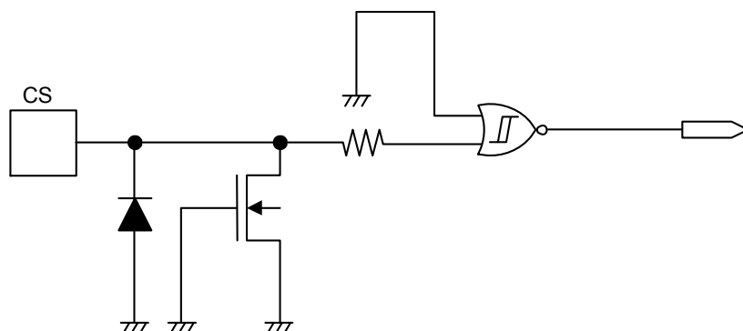
图21 CS端子
