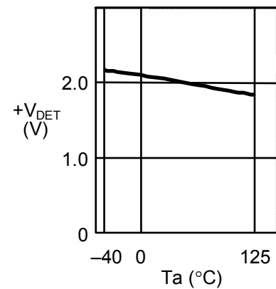
1. 36 低电源解除电压 +V_{DET} —周围温度 T_a
