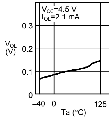
1. 20 低电位输出电压V OL —周围温度Ta
