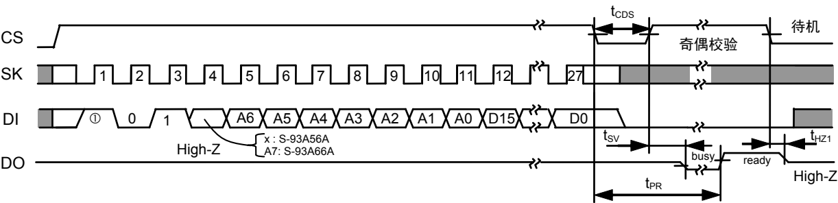
图9 数据写入定时 (S-93A56A, S-93A66A)
