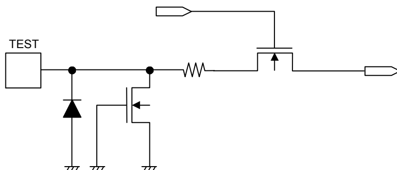
图24 TEST端子
