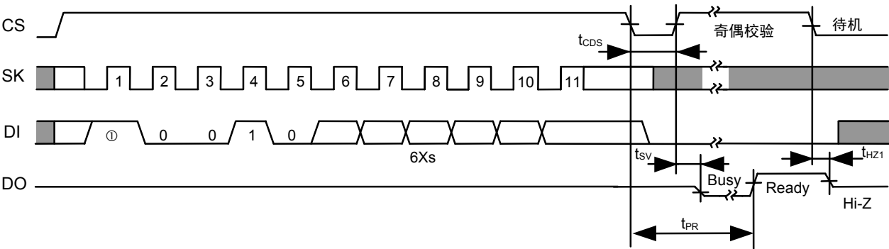
图15 全部删除定时 (S-93A56A, S-93A66A)
