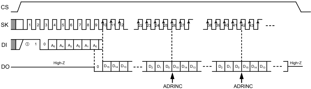
图6 读出定时 (S-93A46A)
