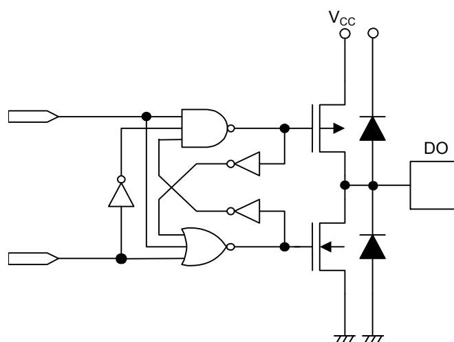
图25 DO端子
