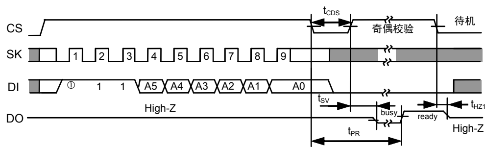
图 10 数据删除定时 (S-93A46A)
