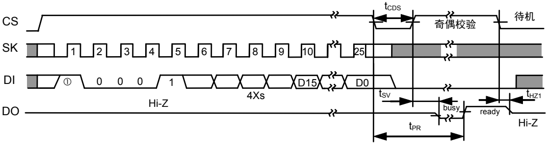
图12 全部写入定时 (S-93A46A)
