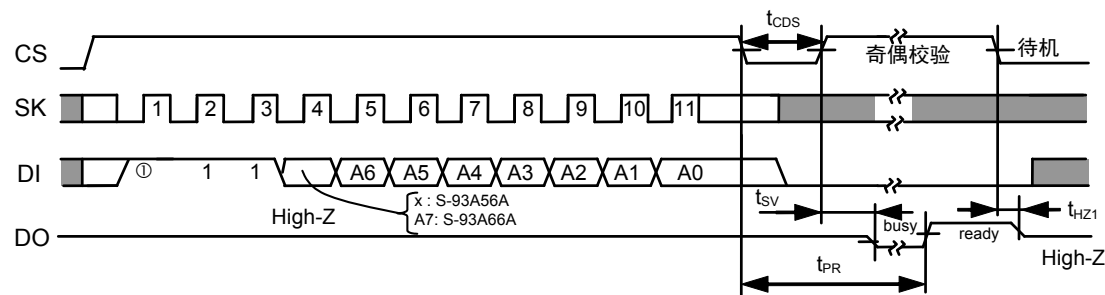
图 11 数据删除定时 (S-93A56A, S-93A66A)
