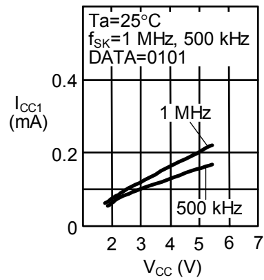
1.4 读出时消耗电流 I_{CC1} —电源电压 V_{CC}
