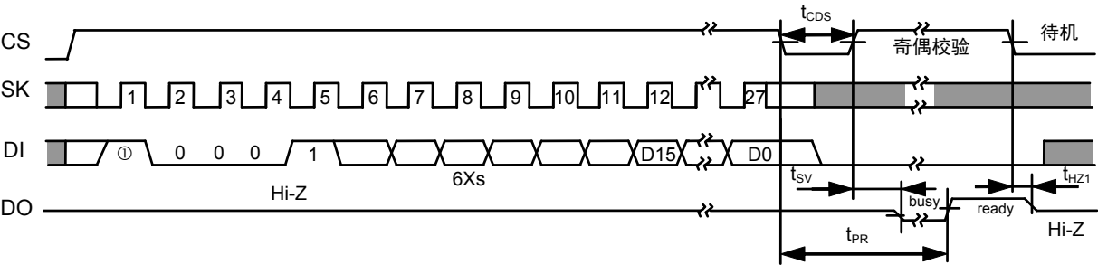
图13 全部写入定时 (S-93A56A, S-93A66A)
