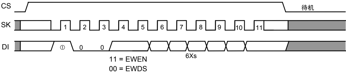
图17 允许或禁止写入定时 (S-93A56A, S-93A66A)
