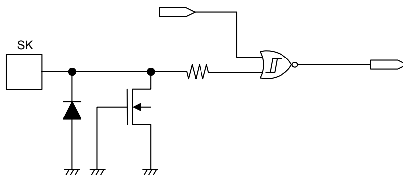
图22 SK端子
