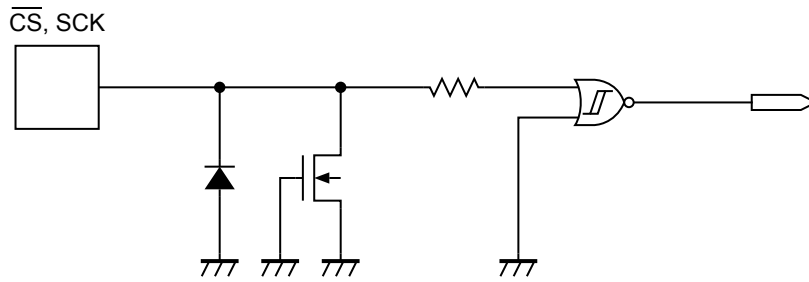
图 22 \overline{\text{CS}} , SCK 端子
