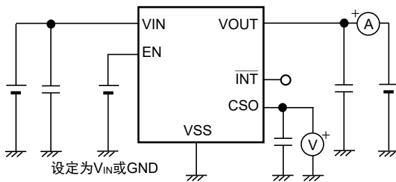
图7 测定电路3
