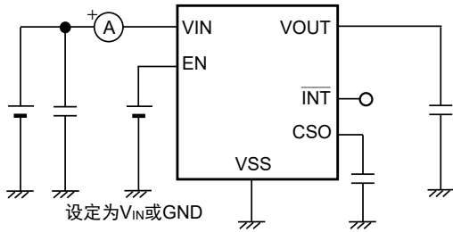
图5 测定电路1
