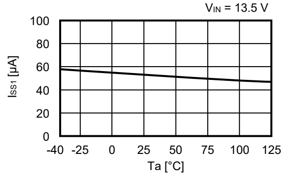
2. 工作时消耗电流 ( I_{SS1} ) – 温度 ( T_a )
