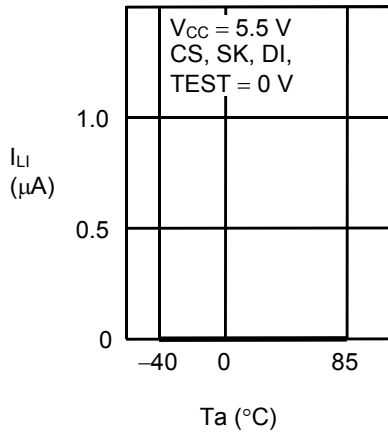
1.13 入力リーク電流 I_{LI} —周囲温度 T_a
