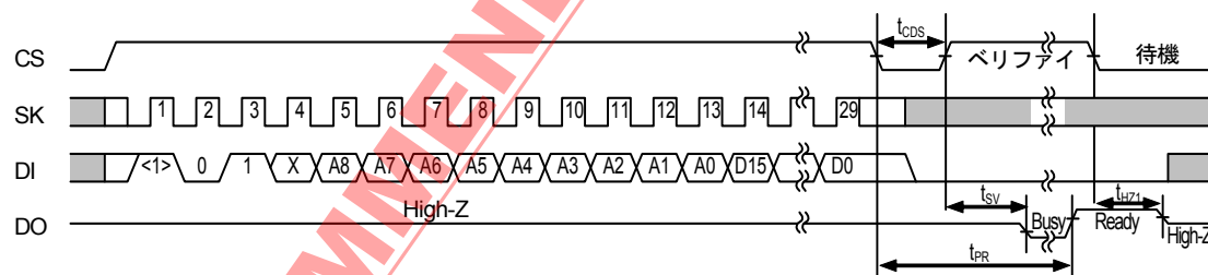
図7 データ書き込みタイミング
