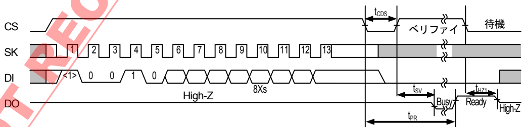
図10 チップ消去タイミング
