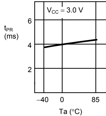
2.4 書き込み時間 t_{PR} —周囲温度 T_a
