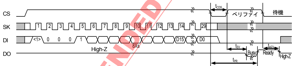
図9 チップ書き込みタイミング
