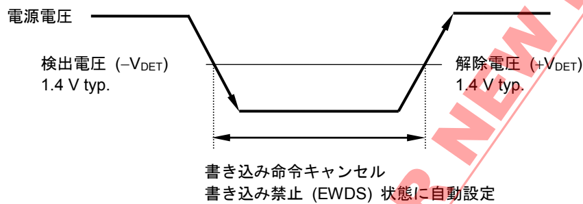
図12 低電源電圧時の動作
