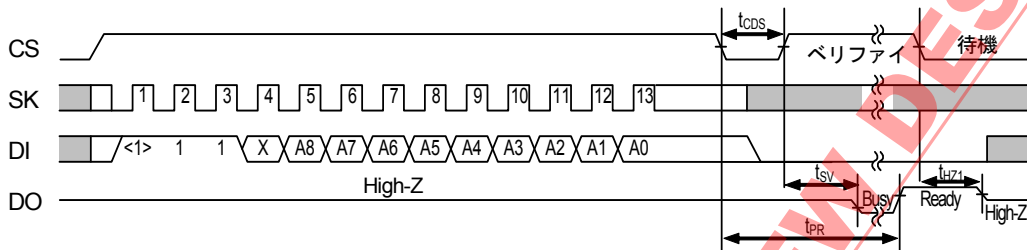
図8 データ消去タイミング
