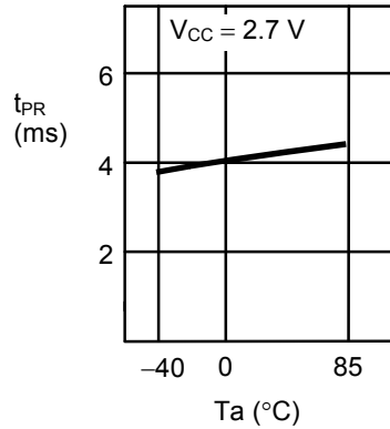
2.5 書き込み時間 t_{PR} —周囲温度 T_a
