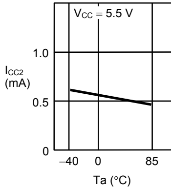
1.7 プログラム時消費電流 I_{CC2} —周囲温度 T_a
