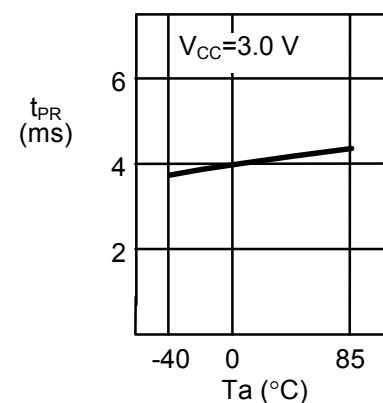
2.4 書き込み時間 t_{PR} —周囲温度 T_a
