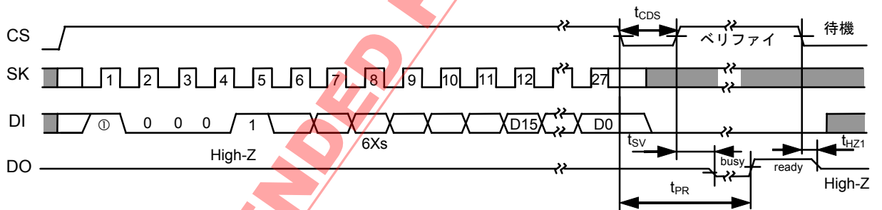
図15 チップ書き込みタイミング (S-93L56A, S-93L66A)
