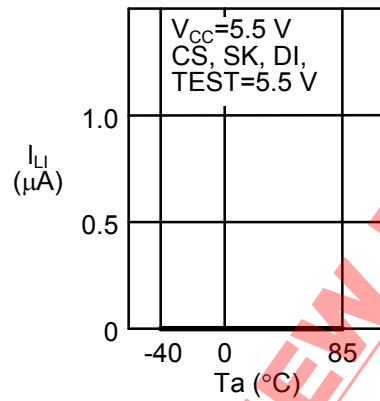
1.14 入力リーク電流 I_{LI} —周囲温度 T_a
