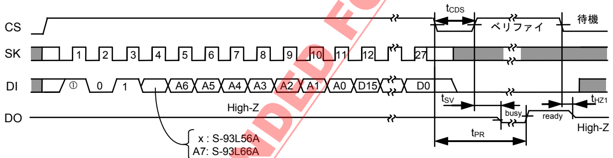
図11 データ書き込みタイミング (S-93L56A, S-93L66A)
