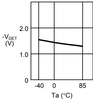
1.31 低電源検出電圧 -V_{DET} —周囲温度 T_a
