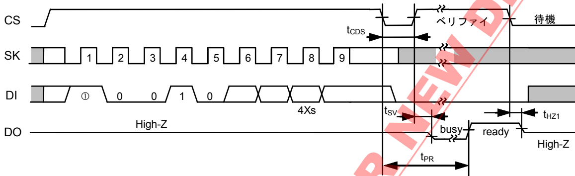
図16 チップ消去タイミング (S-93L46A)
