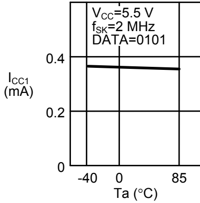
1.1 リード時消費電流 I_{CC1} —周囲温度 T_a
