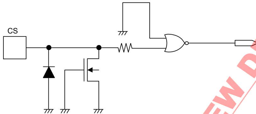
図23 CS端子
