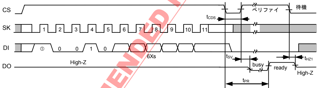
図17 チップ消去タイミング (S-93L56A, S-93L66A)
