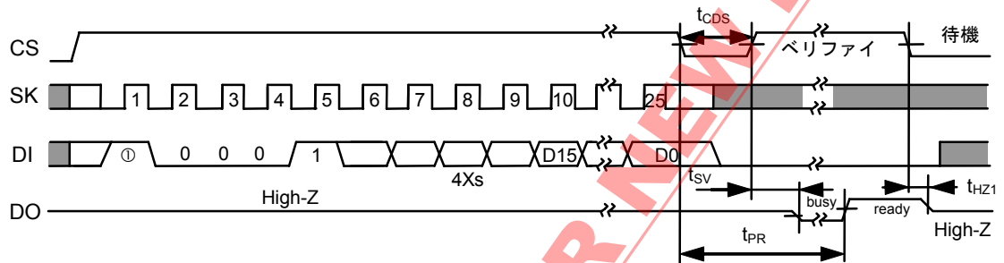
図14 チップ書き込みタイミング (S-93L46A)
