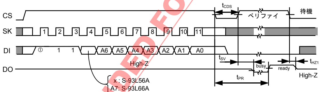
図13 データ消去タイミング (S-93L56A, S-93L66A)
