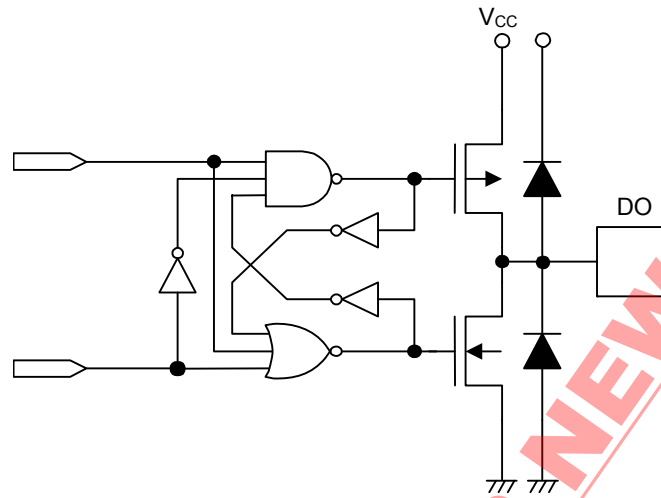
図26 DO端子
