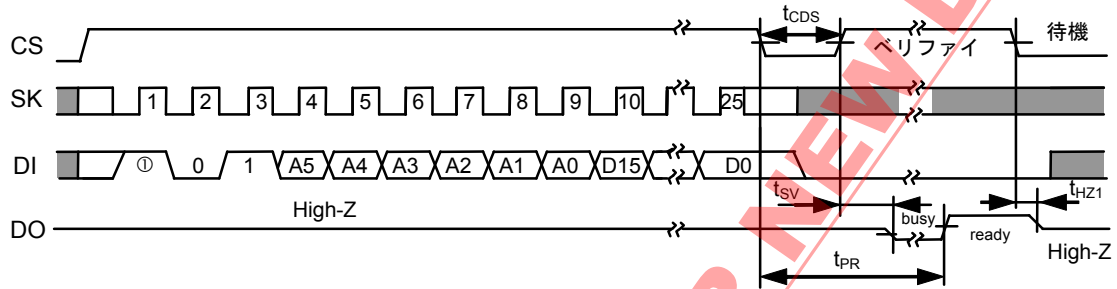
図10 データ書き込みタイミング (S-93L46A)
