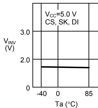
1. 30 入力反転電圧 V_{INV} —周囲温度 T_a
