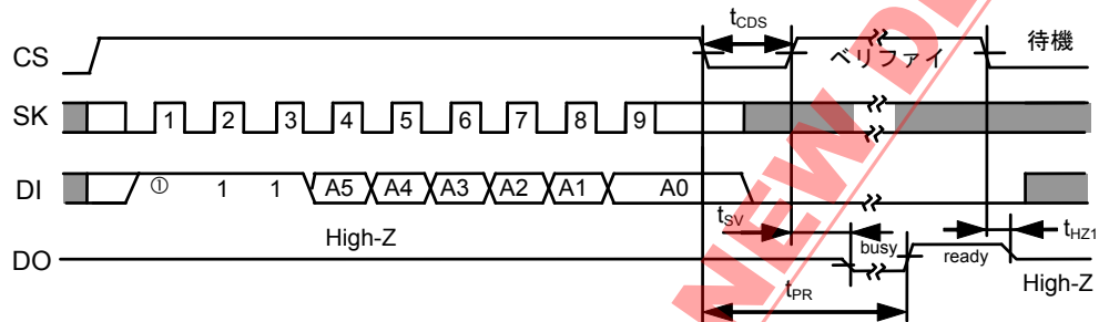
図12 データ消去タイミング (S-93L46A)
