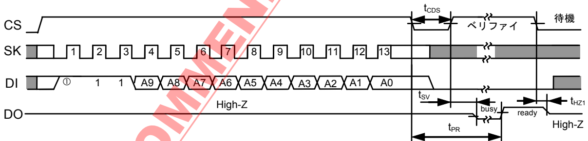
図7 データ消去タイミング
