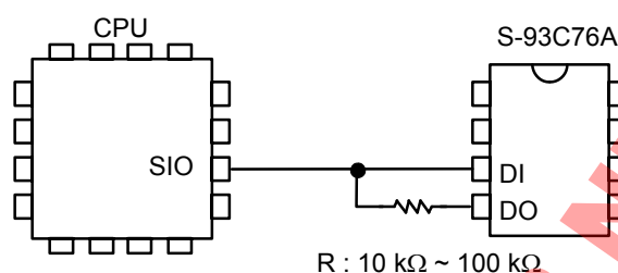
図13 3線式インタフェースの接続法
