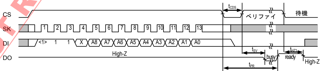
図8 データ消去タイミング
