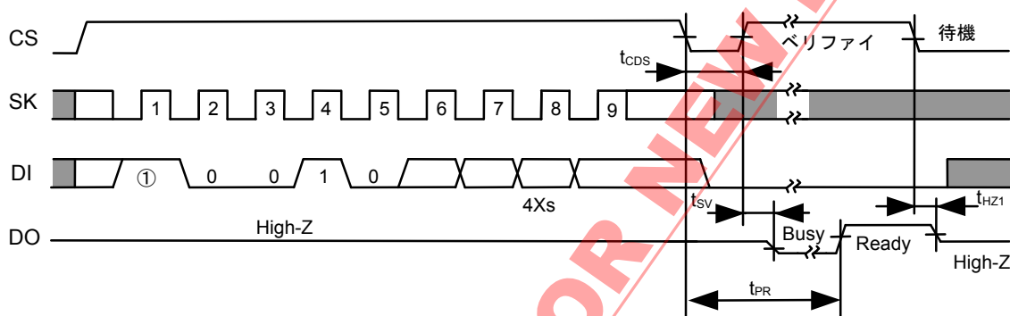
図14 チップ消去タイミング (S-93A46A)
