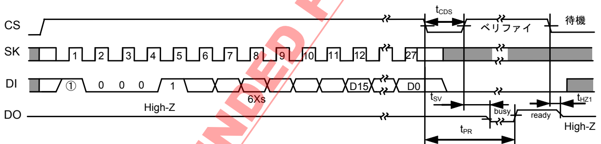
図13 チップ書き込みタイミング (S-93A56A, S-93A66A)
