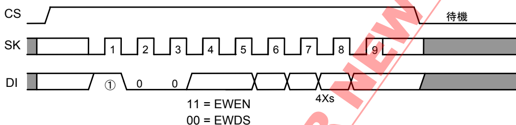
図 16 書き込み許可 / 禁止タイミング (S-93A46A)
