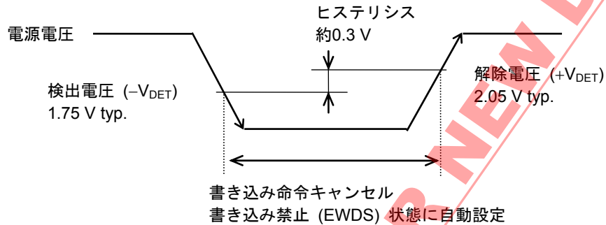
図 18 低電源電圧時の動作
