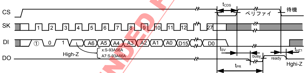
図9 データ書き込みタイミング (S-93A56A, S-93A66A)
