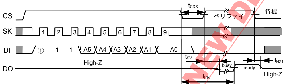
図10 データ消去タイミング (S-93A46A)
