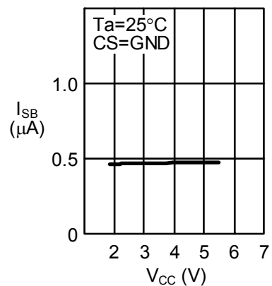
1.12 待機時消費電流 I_{SB} —電源電圧 V_{CC}
