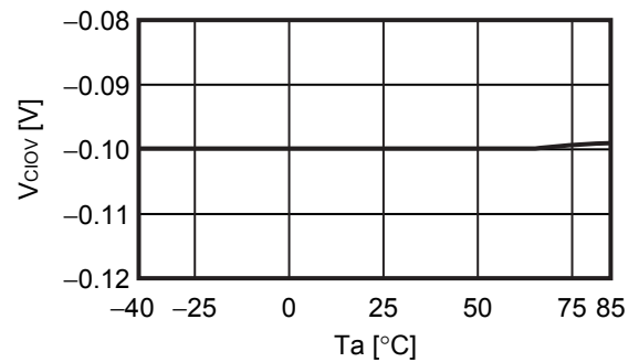
2.16 V_{CIOV} - T_a
