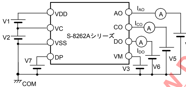
図7 測定回路4
