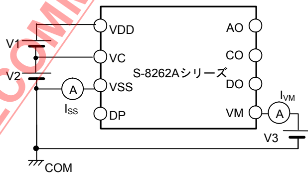
図6 測定回路3
