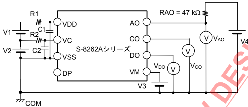
図4 測定回路1
