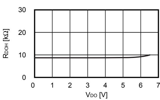
3.3 R_{DOH} - V_{DO}
