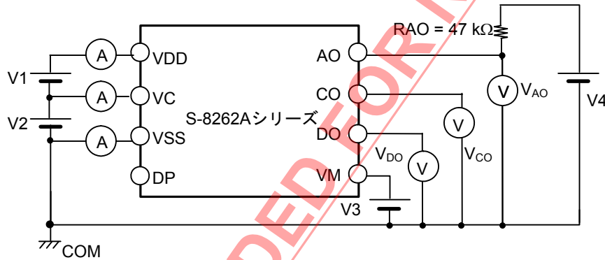
図5 測定回路2
