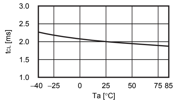
2.6 t_{CL} - T_a
