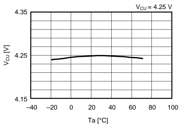
過充電検出電圧 温度依存性
