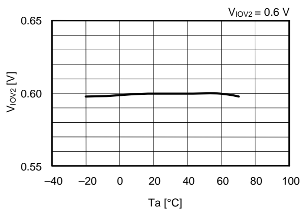
過電流2検出電圧 温度依存性
